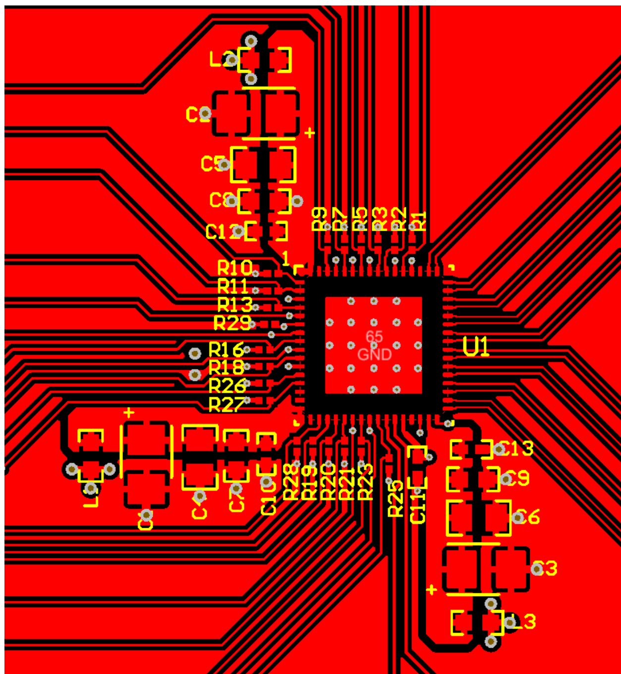
图 11-1. Layout Example
