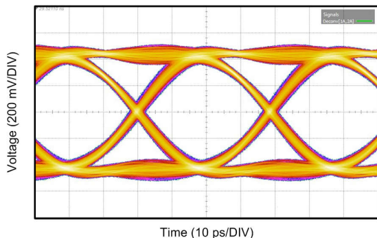
图 7-6. DS280DF810 Operating at 25.78125Gbps
