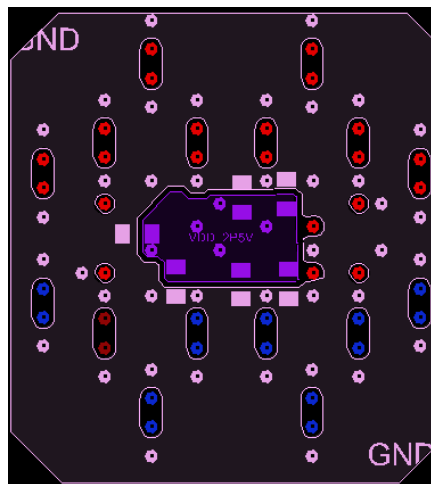
图 7-11. Bottom Layer
