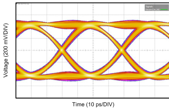
图 18. DS250DF410 Operating at 25.78125 Gbps
