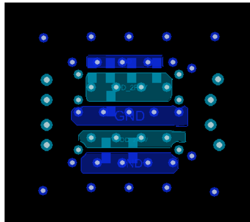
图 29. Bottom Layer
