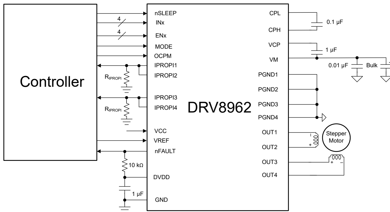
图 8-4. 使用 DRV8962 驱动步进电机
