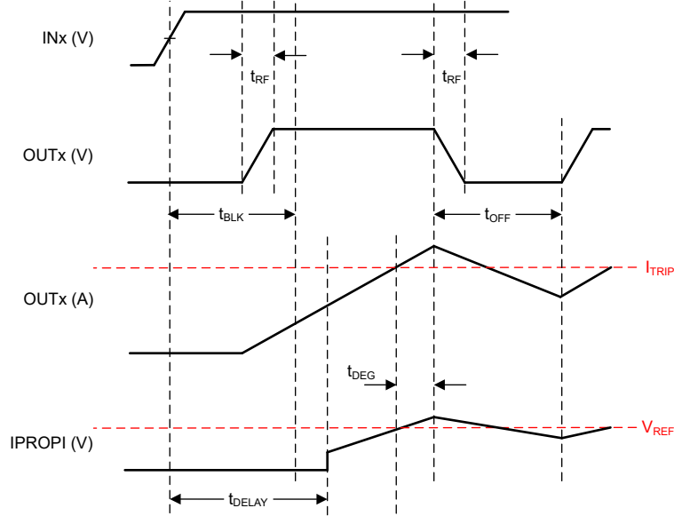
图 6-1. IPROPI 时序图
