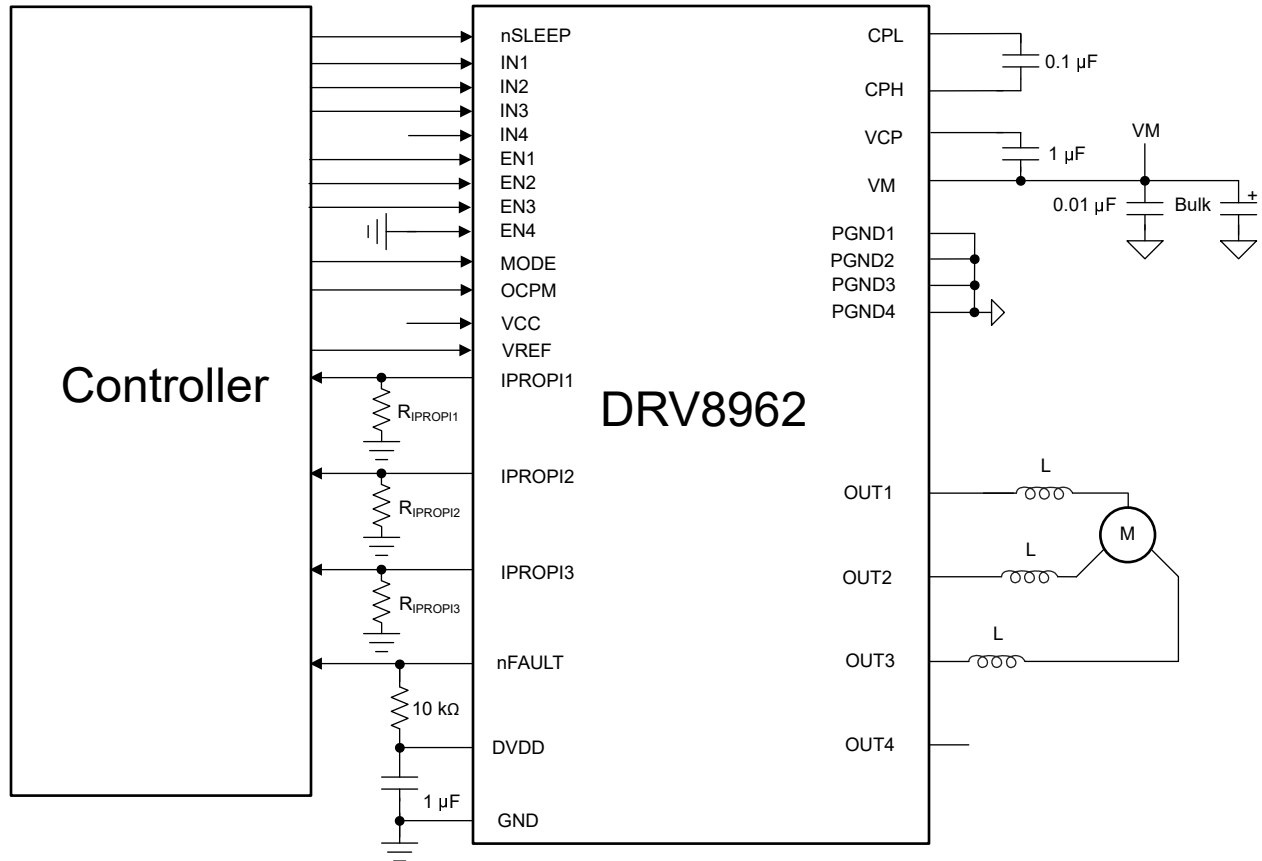
图 8-10. 使用 DRV8962 驱动 BLDC 电机
