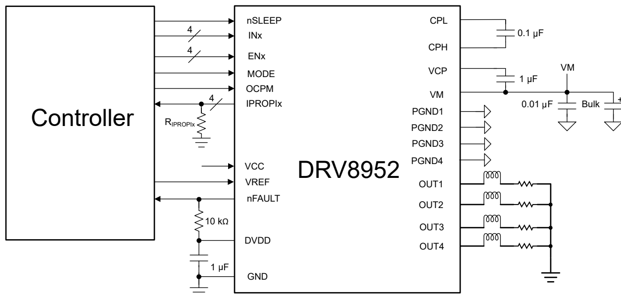
图 7-1. 使用 DRV8952 驱动螺线管
