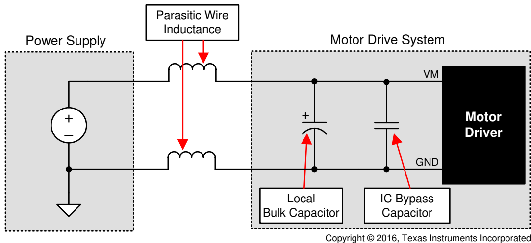
图 7-11. 带外部电源的系统设置示例
