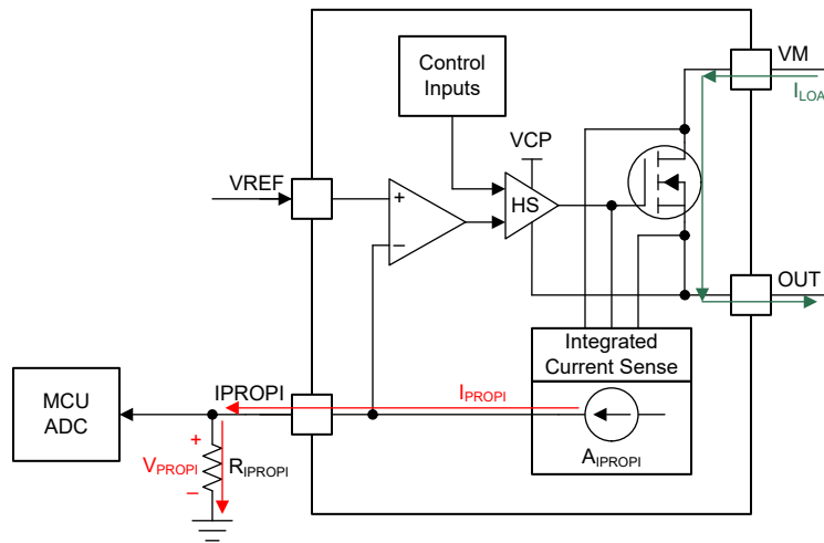
图 6-1. 集成电流检测
