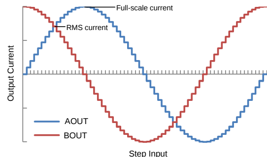
微步进电流波形
