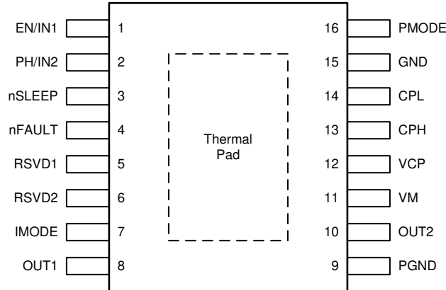
图 5-1. DRV8876N PWP 封装 16 引脚 HTSSOP (带有外露散热焊盘) 顶视图
