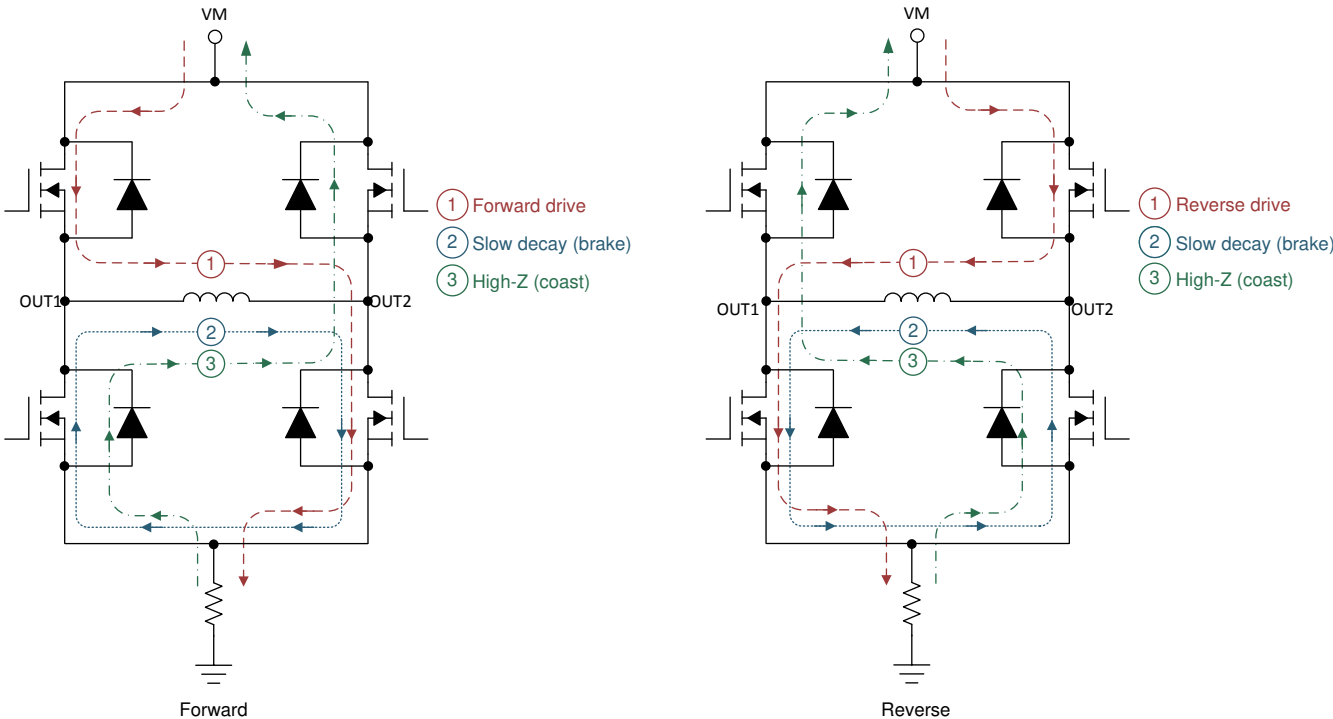
图 7-1. H 桥状态
