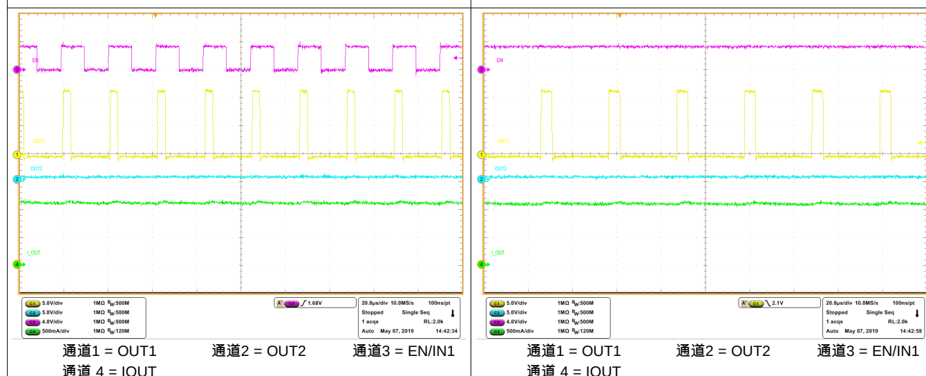
图 28. 带电流斩波的驱动器 PWM 运行
