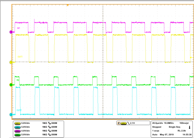
图 8-16. 独立半桥 PWM 运行
