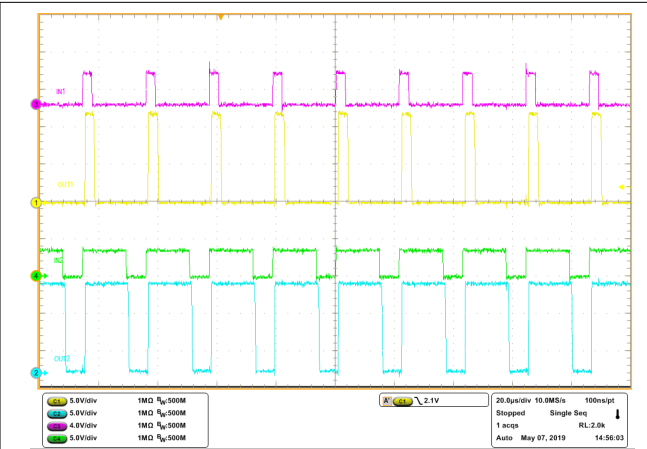
图 8-17. 独立半桥 PWM 运行
