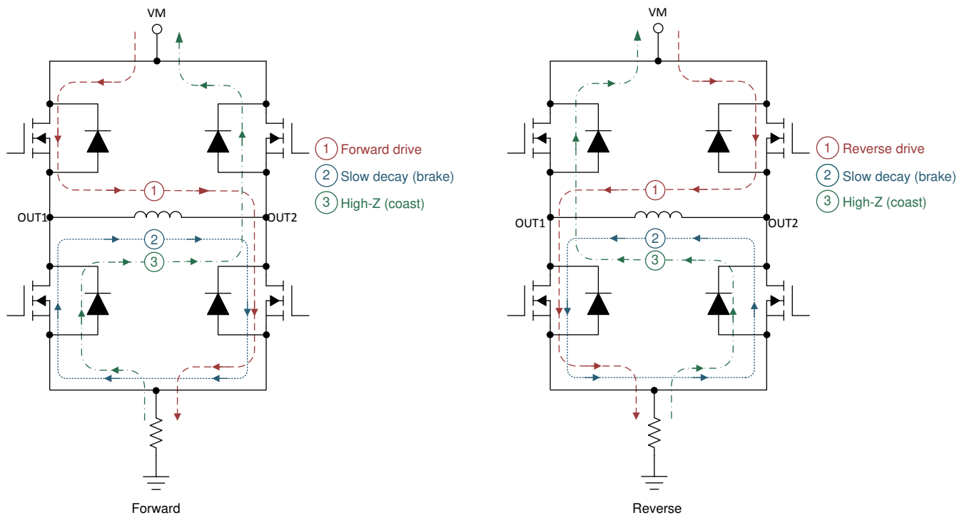
图 7-1. H 桥状态
