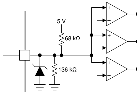
图 7-9. 四电平输入
