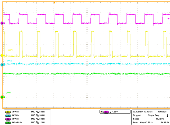
图 8-13. 带电流斩波的驱动器 PWM 运行
