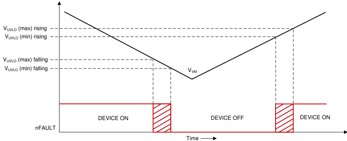
图 7-19. VM UVLO 运行
