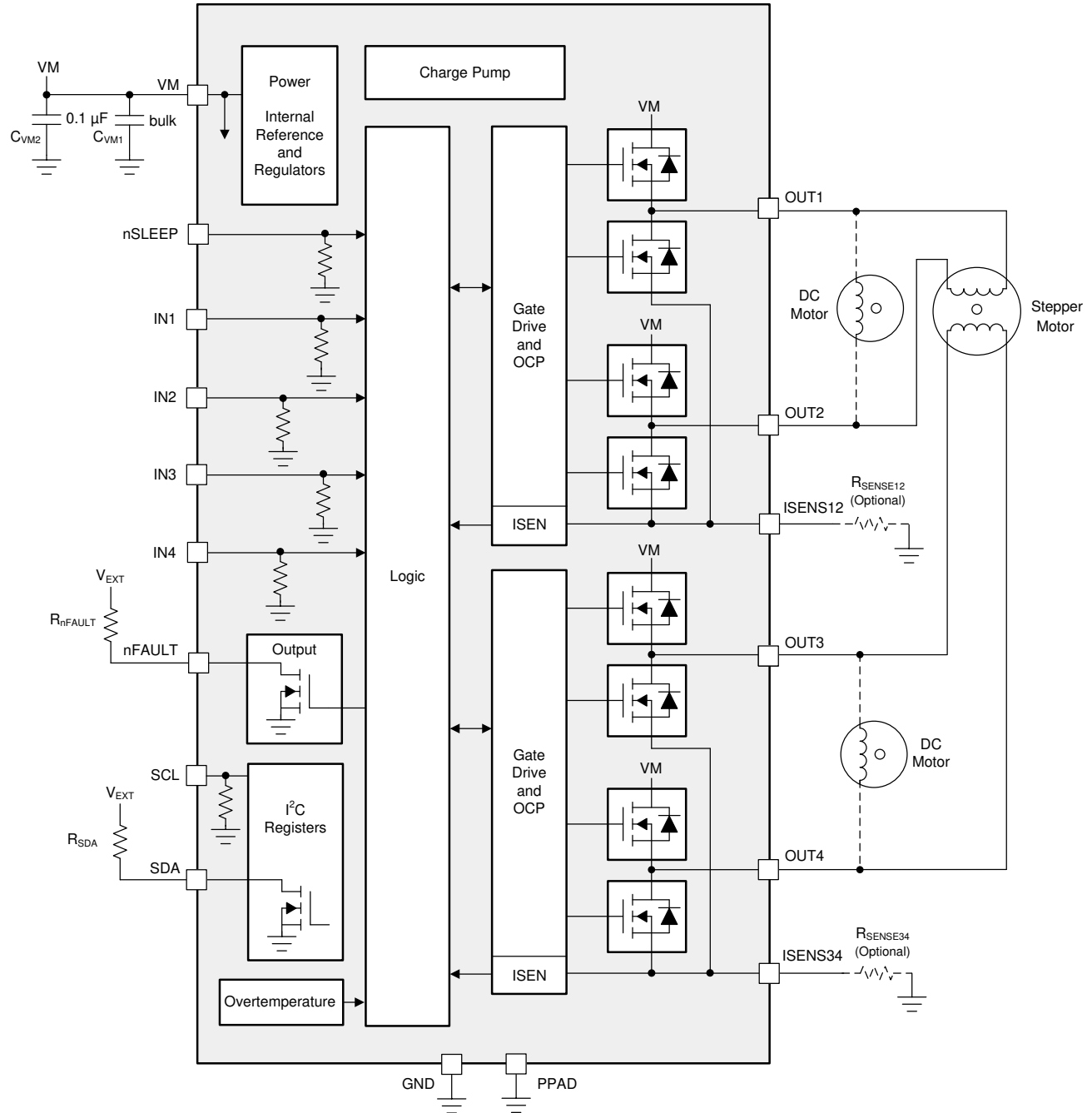
图 7-2. DRV8847S 的方框图
