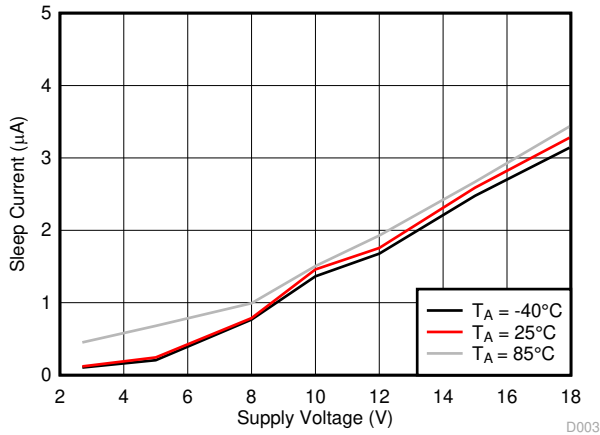
图 6-5. 睡眠模式电源电流 ( I_{VMQ} ) 与电源电压 ( V_{VM} ) 间的关系
