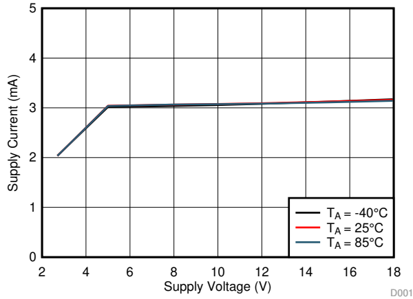
图 6-3. 工作电源电流 ( I_{VM} ) 与电源电压 ( V_{VM} ) 间的关系
