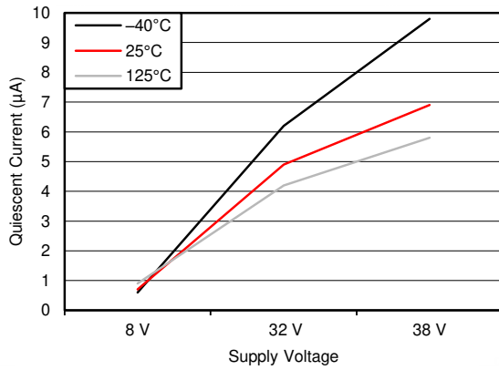
图 6-3. I_{VBBQ} vs V_{BB}
