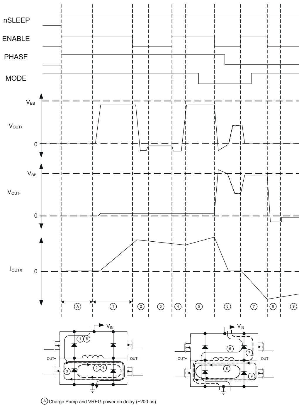
图 7-1. PWM Control Timing
