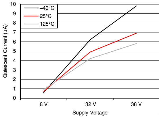
图 6-1. I_{VBBQ} vs V_{BB}
