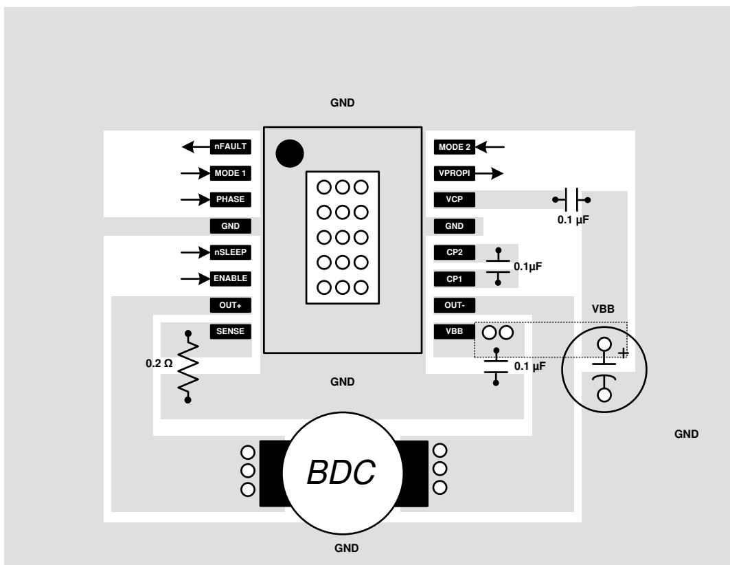
图 11-2. PWP Layout Example
