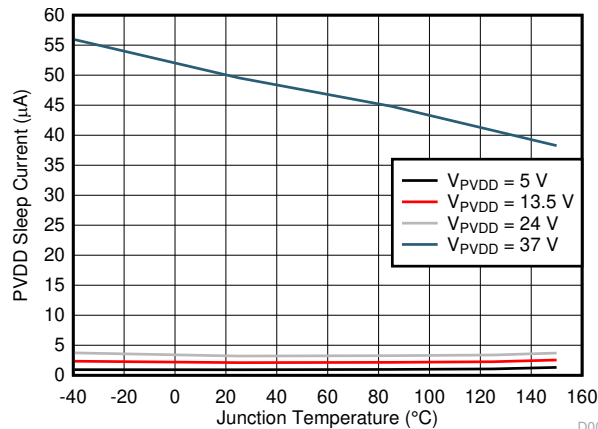
图 6-2. PVDD Sleep Current
