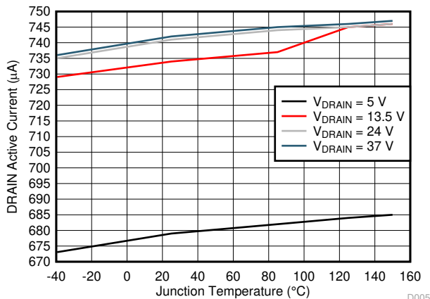
图 6-6. DRAIN Active Current
