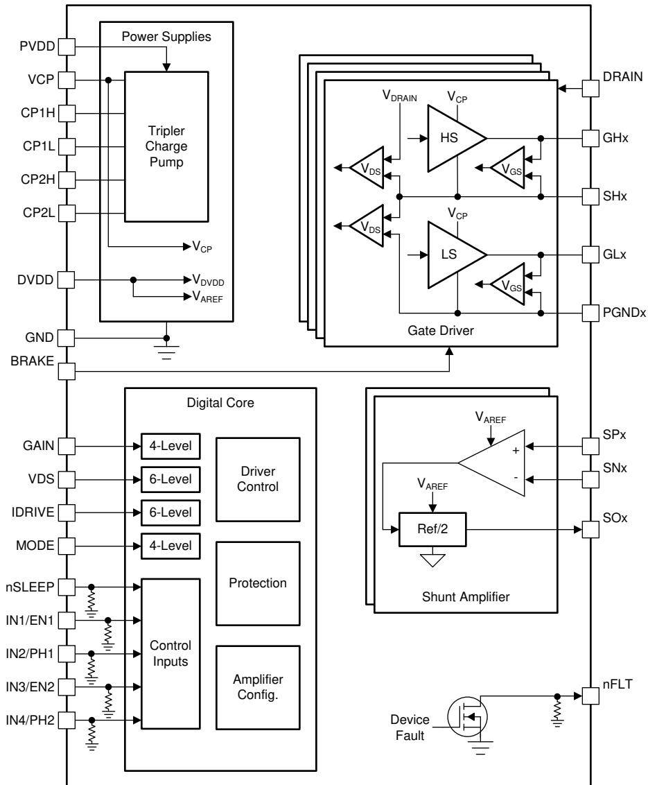
图 7-4. Block Diagram for DRV8714H-Q1 RHA Package
