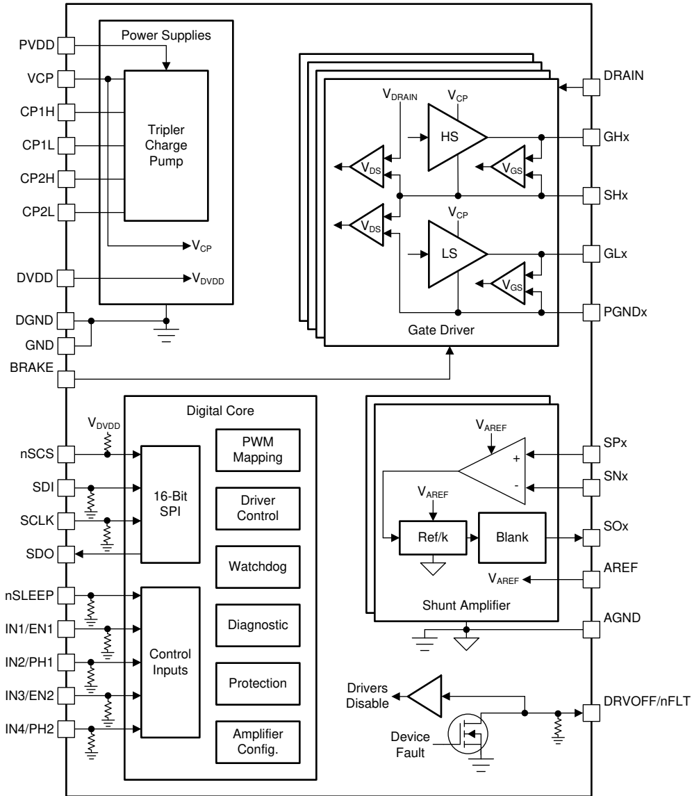
图 7-2. Block Diagram for DRV8714S-Q1 RVJ Package
