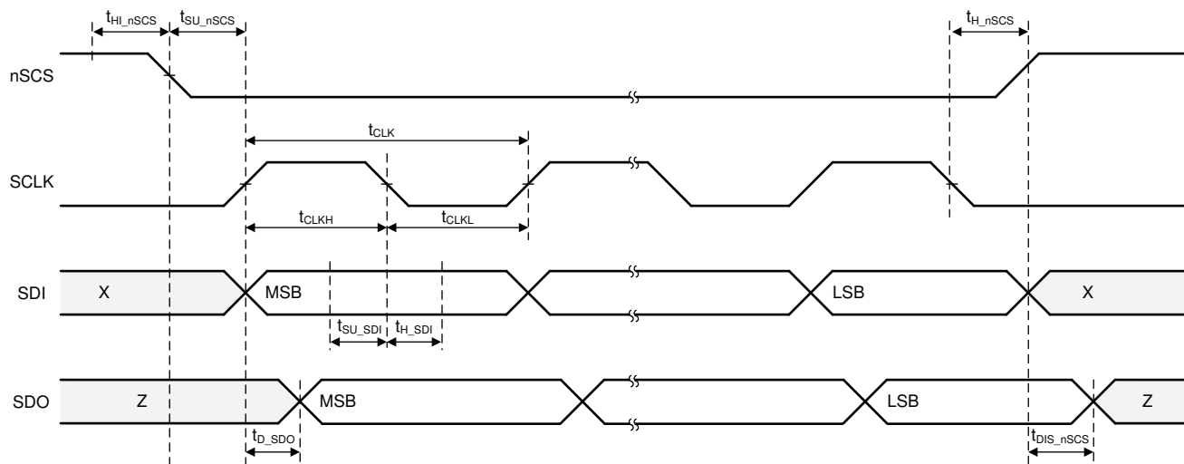
图 6-1. SPI Timing Diagram
