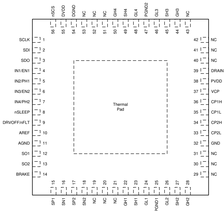
图 5-2. DRV8714S-Q1 VQFN (RVJ) 56-Pin Package Top View
