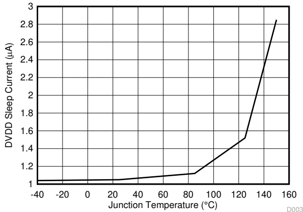
图 6-4. DVDD Sleep Current
