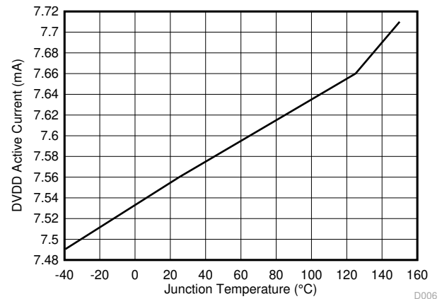
图 6-7. DVDD Active Current
