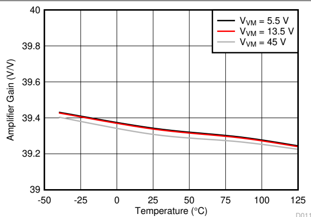
图 6-9. Amplifier Gain
