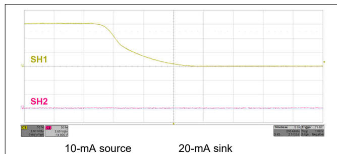
图 8-2. SH1 Fall Time
