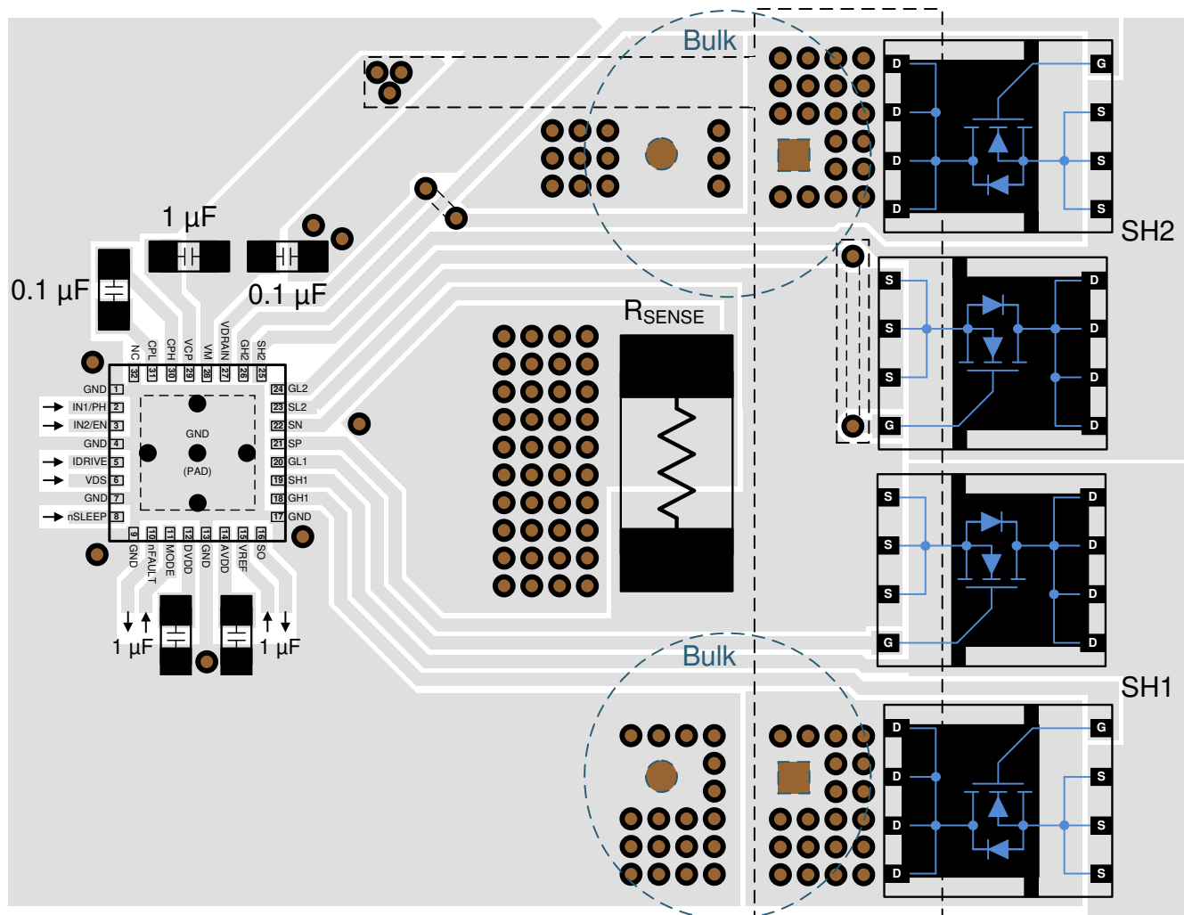
图 10-1. DRV8702-Q1 Layout Example
