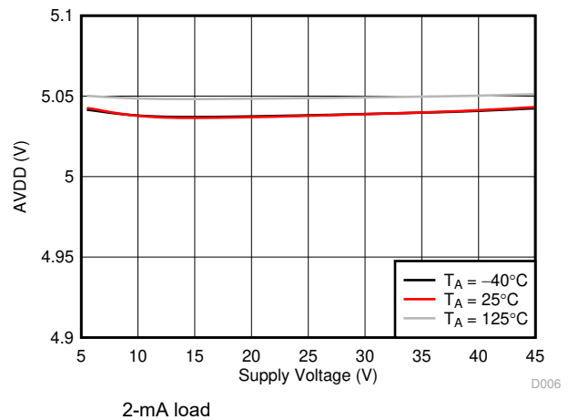
图 6-6. AVDD Regulator
