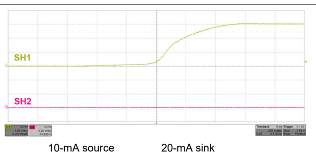
图 8-3. SH1 Rise Time
