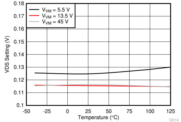
图 6-14. OCP Threshold Voltage
