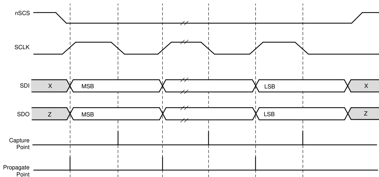
图 7-18. SPI Transaction
