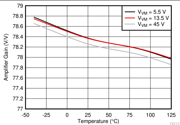
图 6-10. Amplifier Gain
