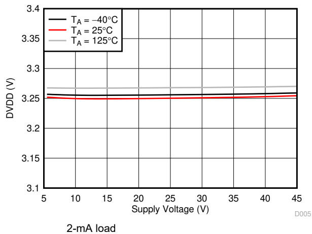
图 6-5. DVDD Regulator
