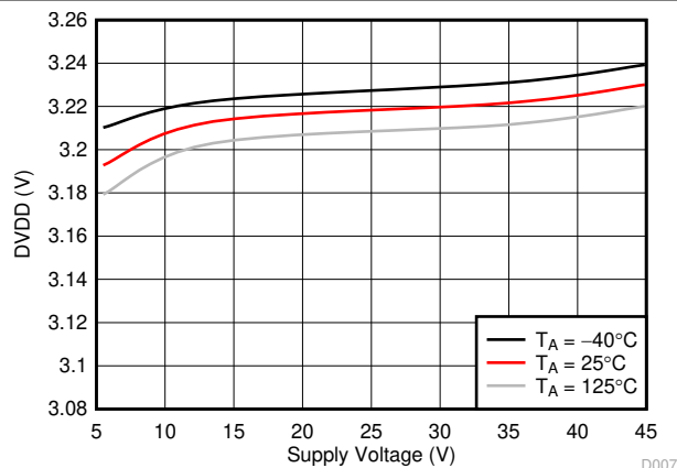
图 6-7. DVDD Regulator
