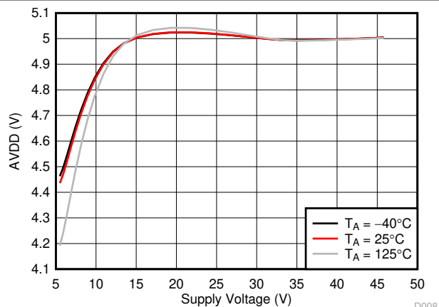
图 6-8. AVDD Regulator
