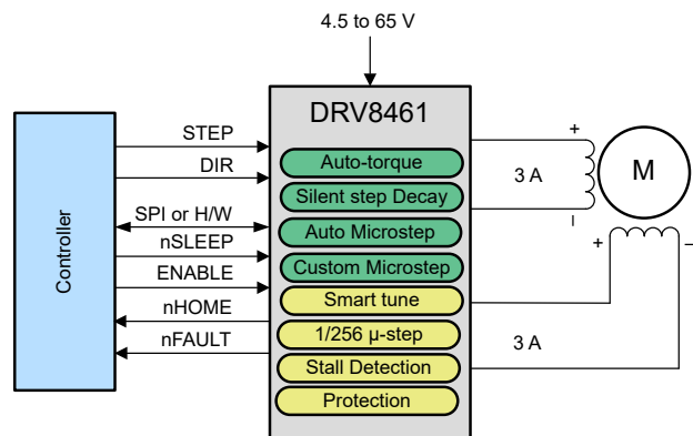
简化原理图
