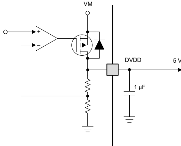
图 7-31. 线性稳压器方框图
