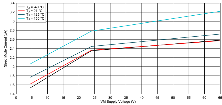
图 6-3. 睡眠模式电源电流
