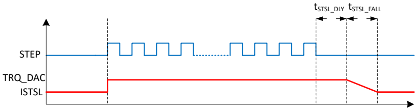
图 7-11. 静止省电模式
