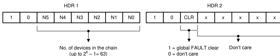
图 7-52. 标头字节
