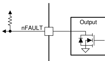
图 7-46. nFAULT 引脚
