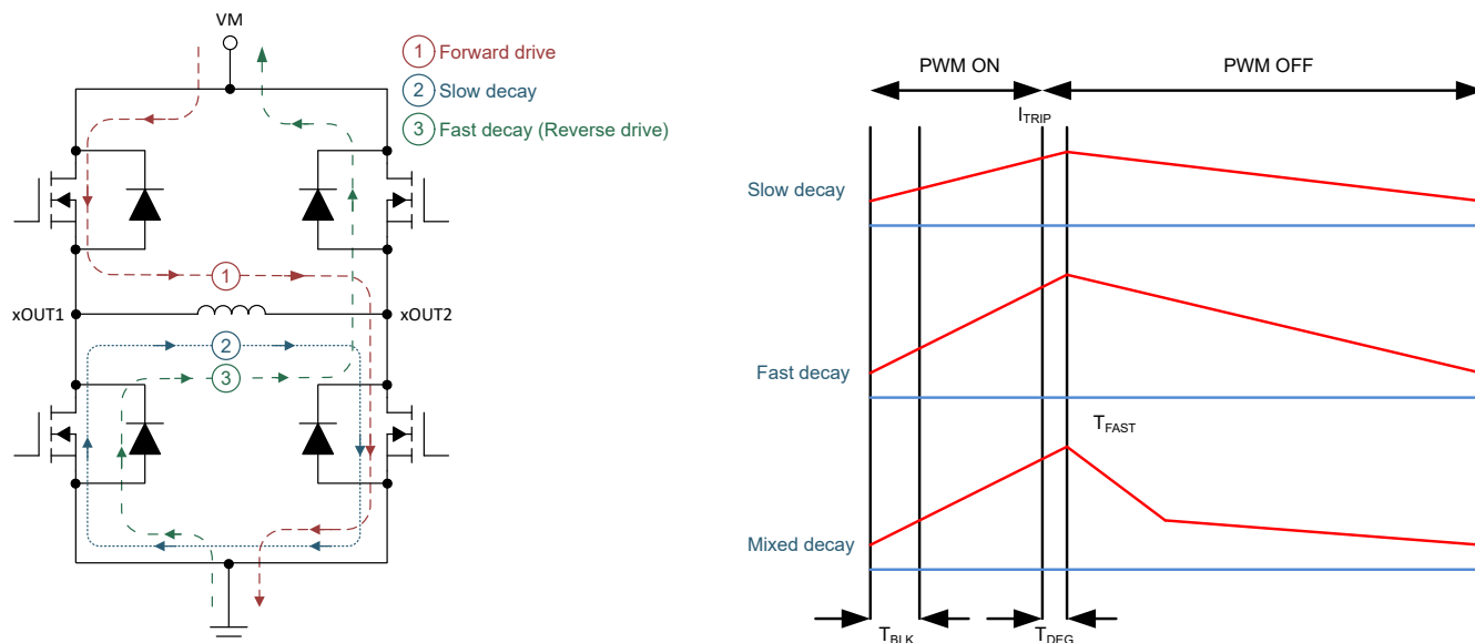
图 7-12. 衰减模式
