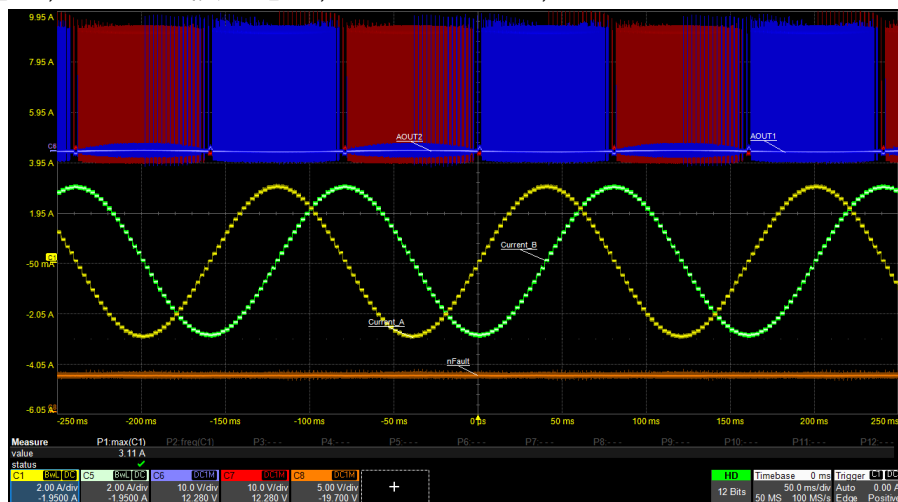
图 8-2. 在 400pps、 I_{FS} = 3 \text{ A} 时为 1/16 微步进
