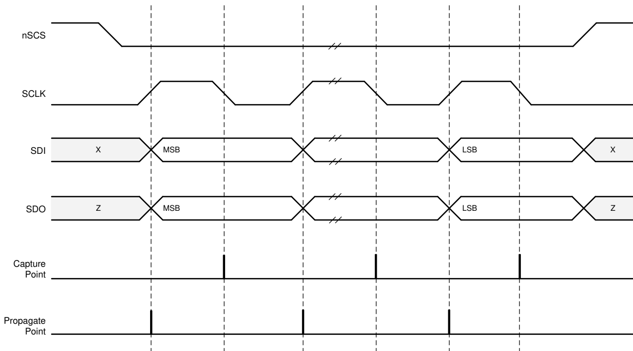
图 7-54. SPI 事务
