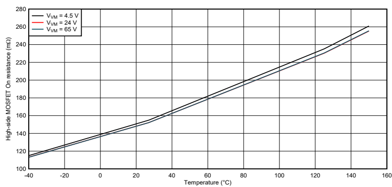
图 6-6. 高侧 FET 导通电阻
