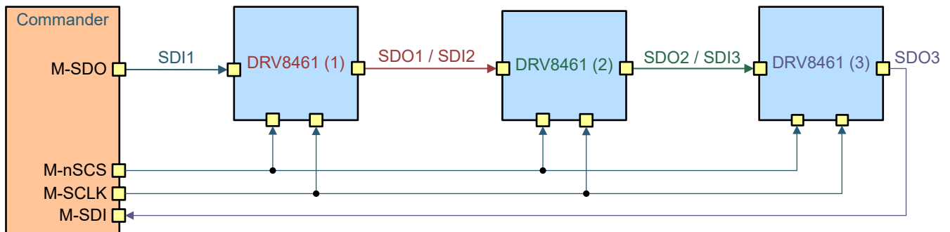
图 7-49. 在菊花链中连接三个器件
