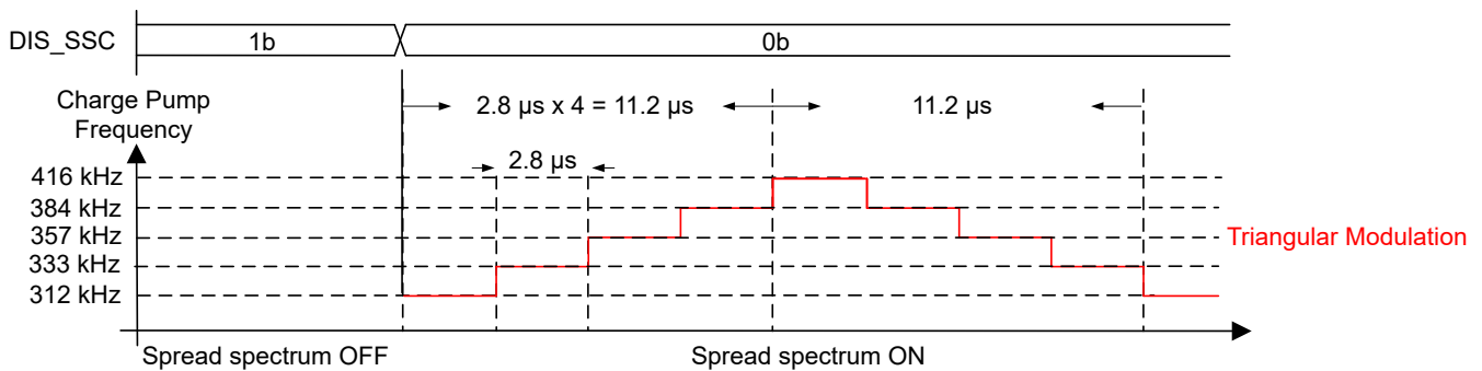
图 7-38. 电荷泵时钟的三角展频
