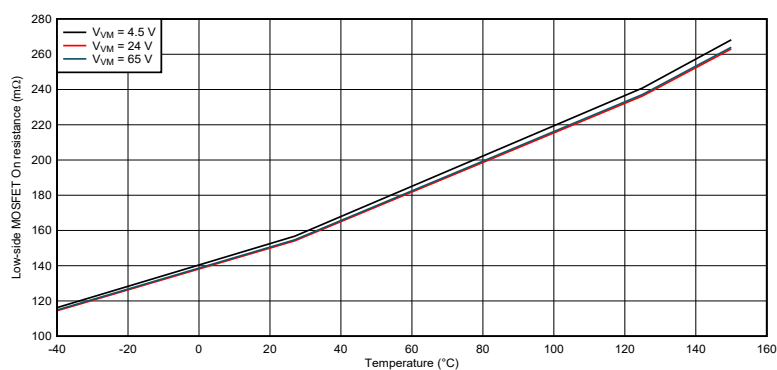
图 6-7. 低侧 FET 导通电阻
