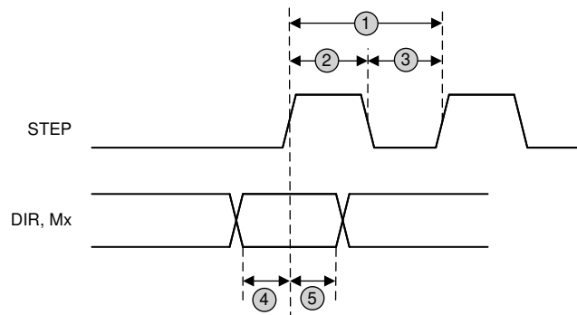
图 6-1. 时序图
