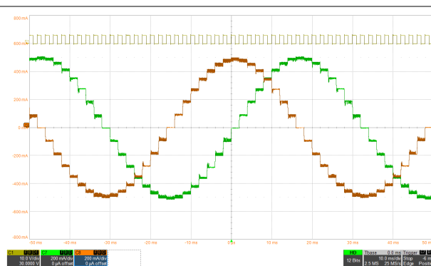
图 8-4. 智能调优动态衰减下的 1/8 微步进
