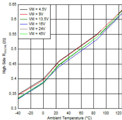
图 6-9. 高侧 R_{DS(on)} 与温度之间的关系
