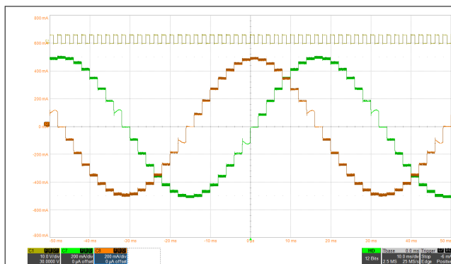
图 8-3. 智能调优纹波控制衰减下的 1/8 微步进
