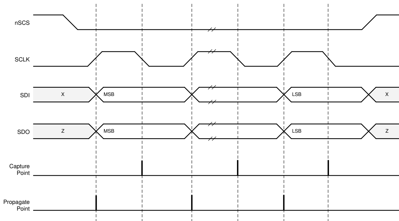
图 7-29. SPI 事务
