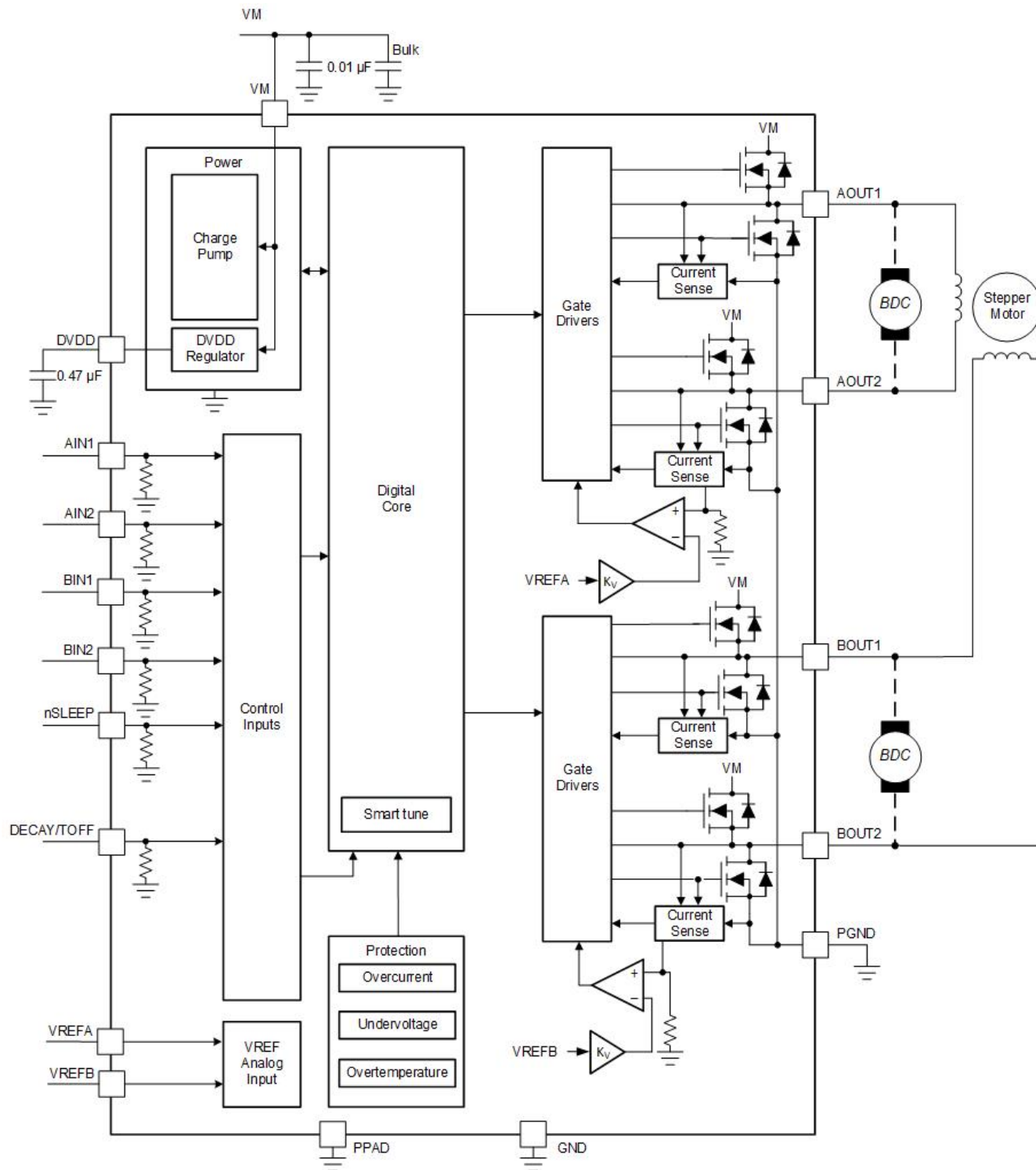
图 7-2. DRV8428P 方框图
