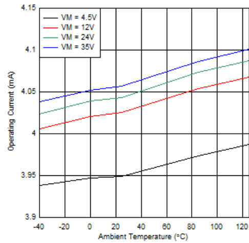
图 6-5. 工作电流与温度间的关系
