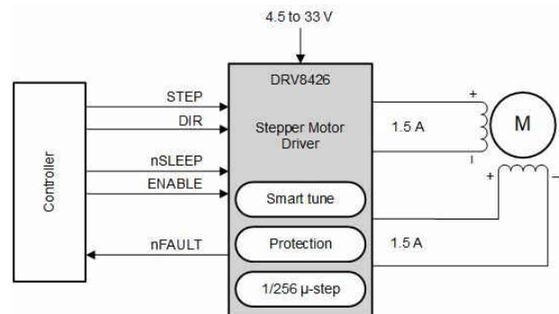
简化原理图
