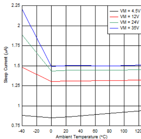
图 6-3. 睡眠电流与温度间的关系
