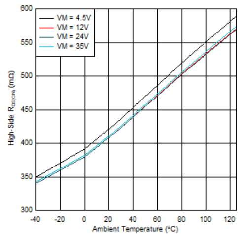
图 6-9. 高侧 R_{DS(ON)} 与温度间的关系
