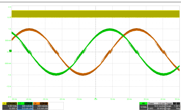
图 8-8. 智能调优动态衰减下的 1/256 微步进
