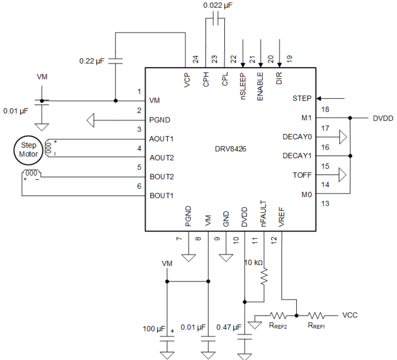
图 8-2. 典型应用原理图 ( 1/8 微步进、智能调优纹波控制衰减、VQFN 封装 )
