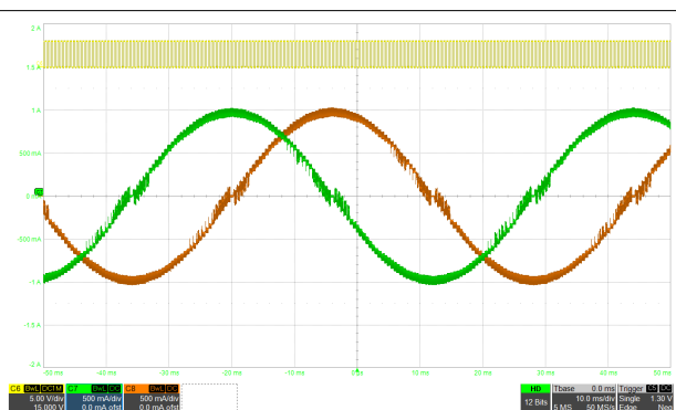
图 8-6. 智能调优动态衰减下的 1/32 微步进
