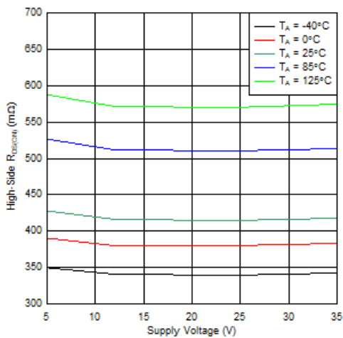
图 6-8. 高侧 R_{DS(ON)} 与电源电压之间的关系
