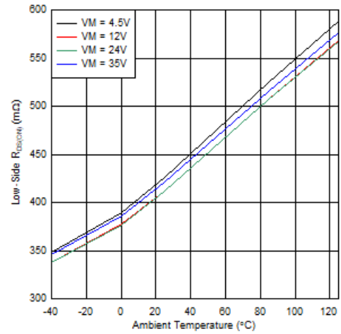
图 6-7. 低侧 R_{DS(ON)} 与温度间的关系
