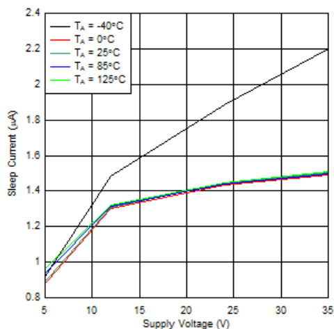
图 6-2. 睡眠电流与电源电压间的关系
