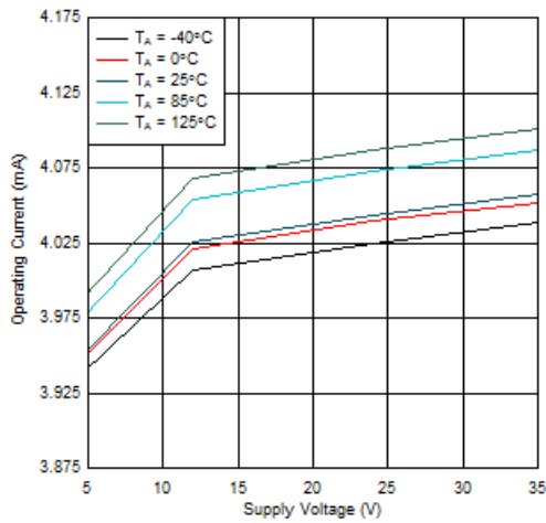
图 6-4. 工作电流与电源电压之间的关系
