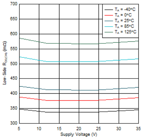
图 6-6. 低侧 R_{DS(ON)} 与电源电压之间的关系
