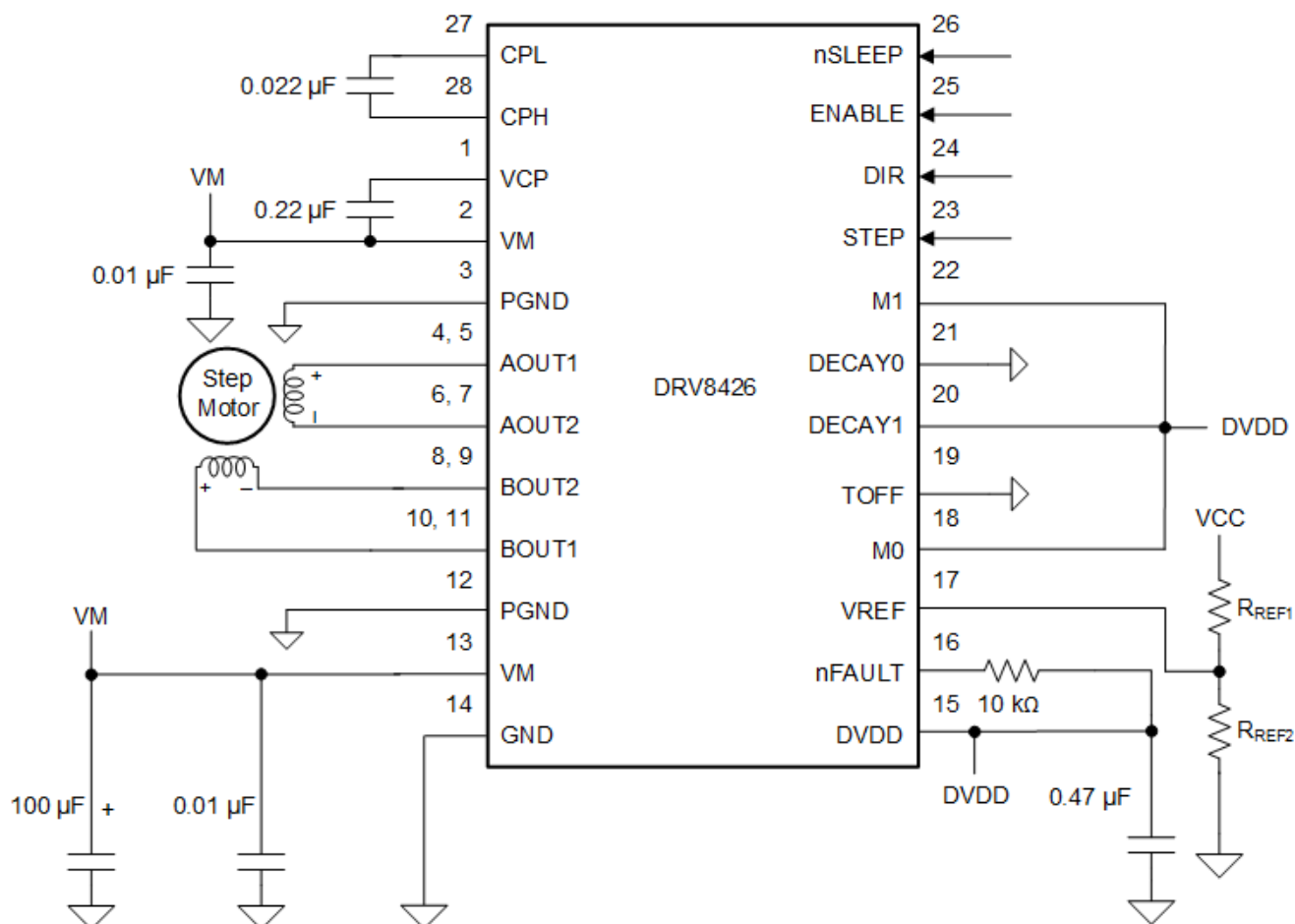
图 8-1. 典型应用原理图 ( 1/8 微步进、智能调优纹波控制衰减、HTSSOP 封装 )
