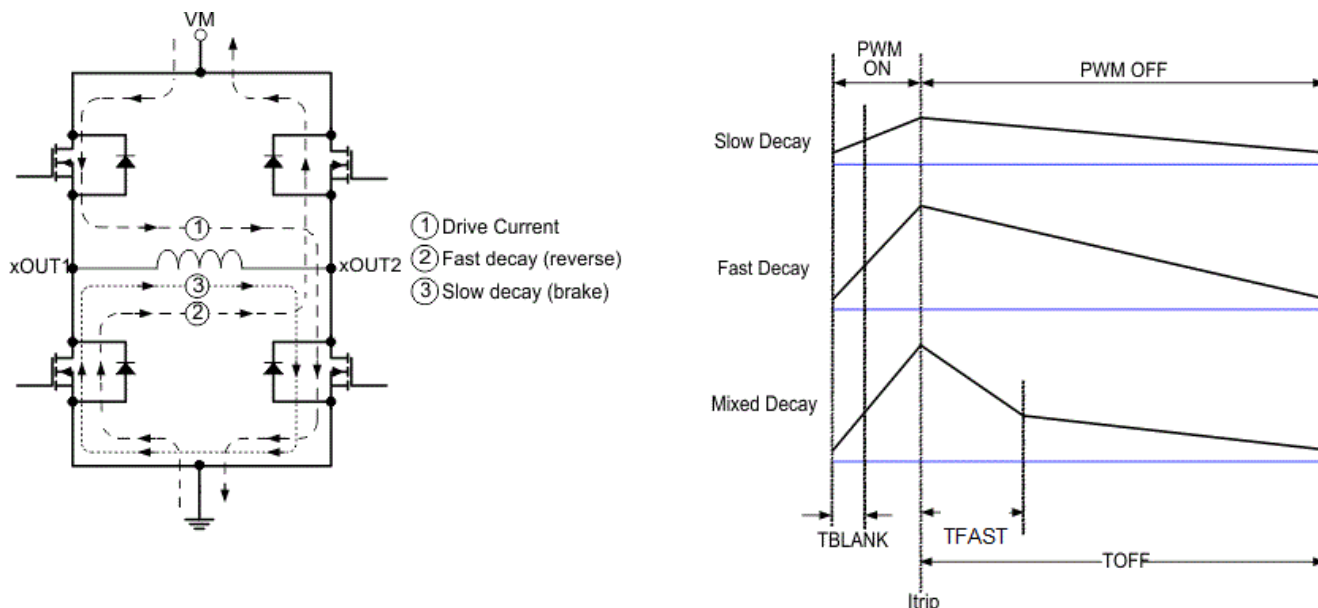
图 7-7. 衰减模式
