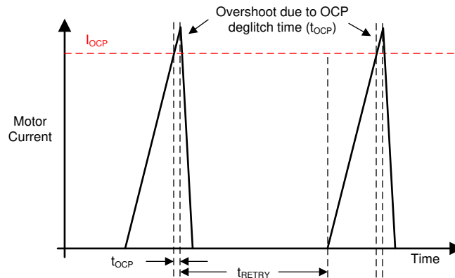
图 8-7. OCP 运行
