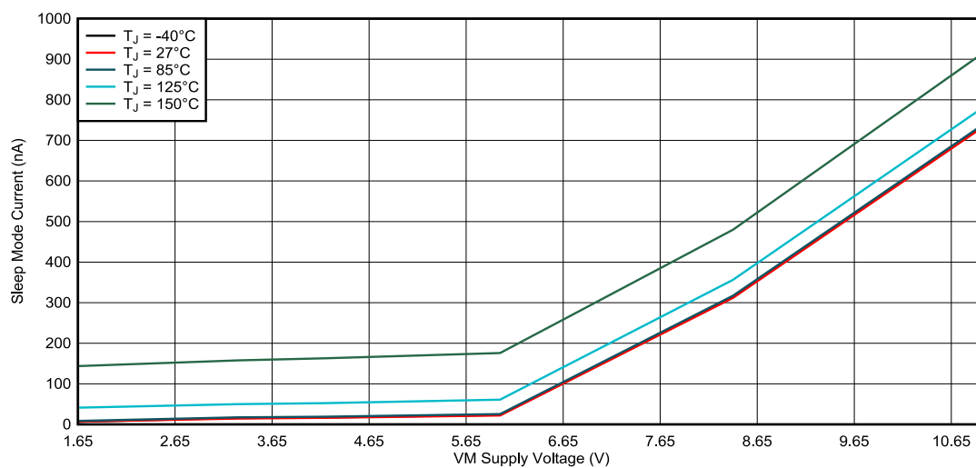
图 7-2. 睡眠模式电流
