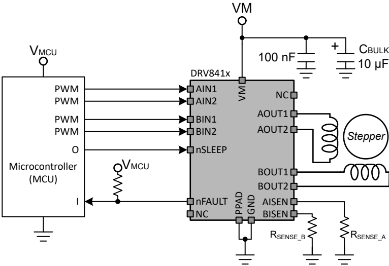
图 9-1. DRV8411 驱动步进电机的典型应用原理图
