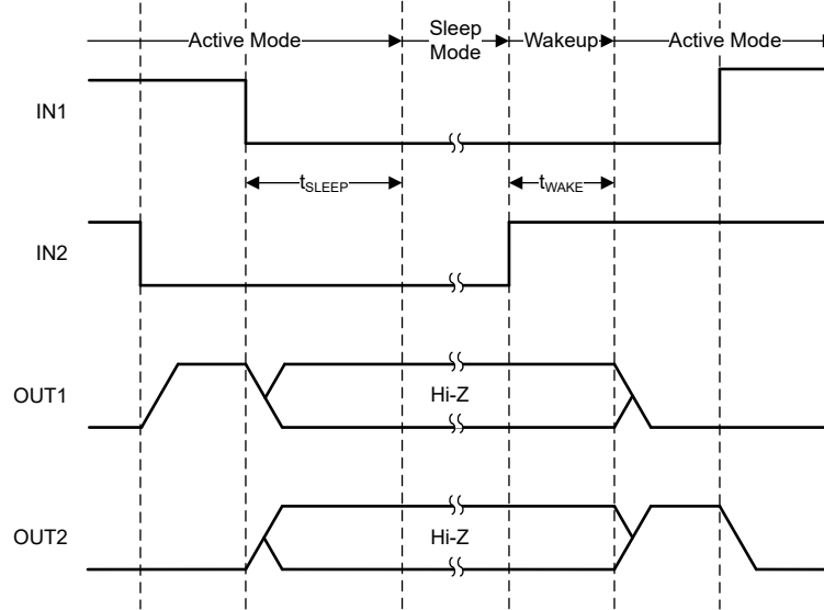
图 8-8. 睡眠模式进入和唤醒时序图
