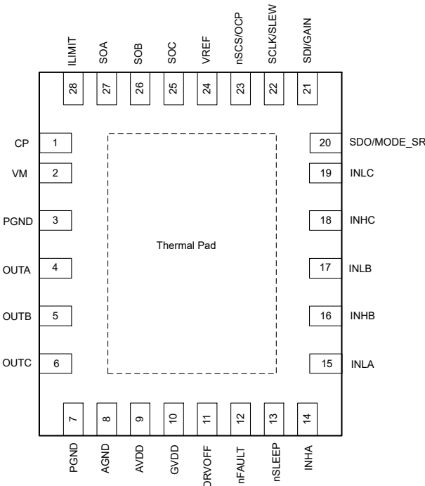
图 5-1. DRV8376 28 引脚 VQFN (带有外露散热焊盘) 顶视图
