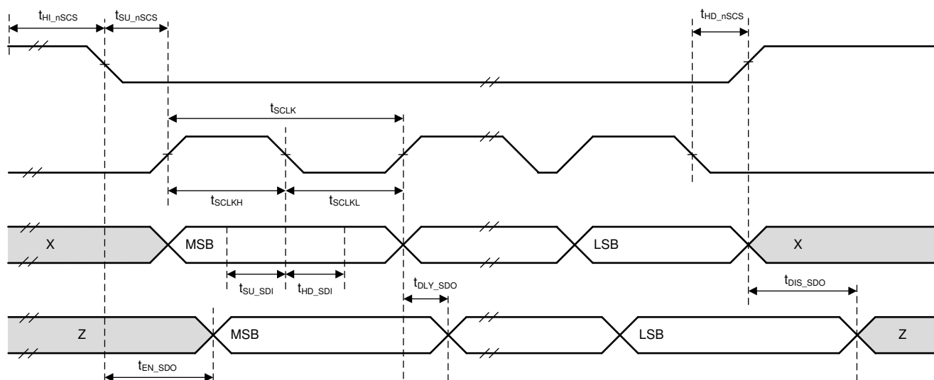
图 6-1. SPI 辅助模式时序
