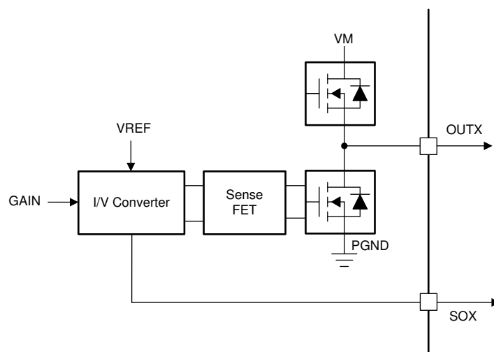
图 7-20. 集成电流检测放大器
