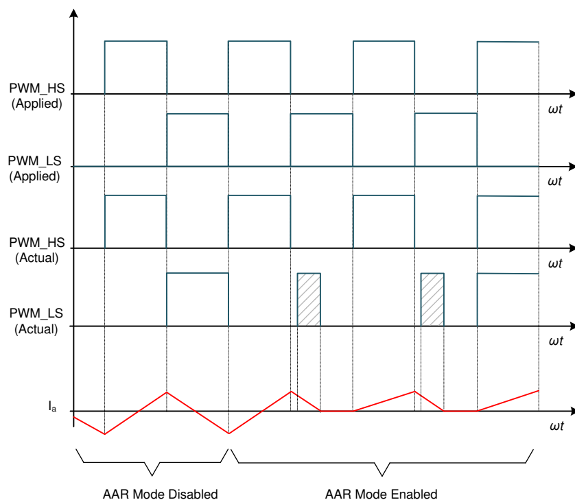
图 7-27. AAR 处于 PWM 模式
