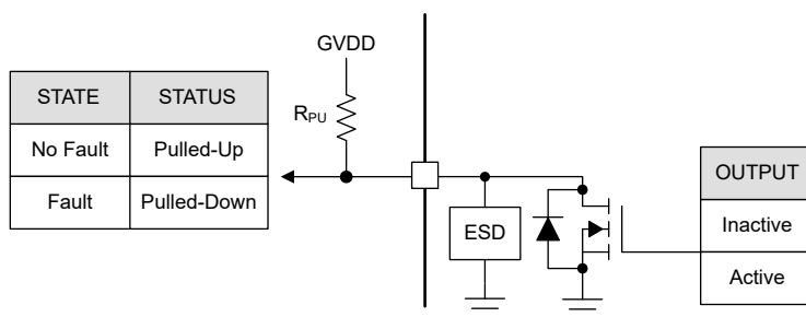
图 7-17. 漏极开路
