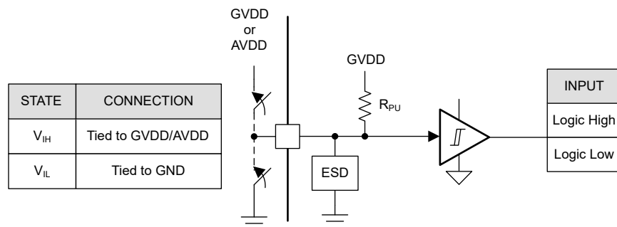
图 7-16. 逻辑 nSCS
