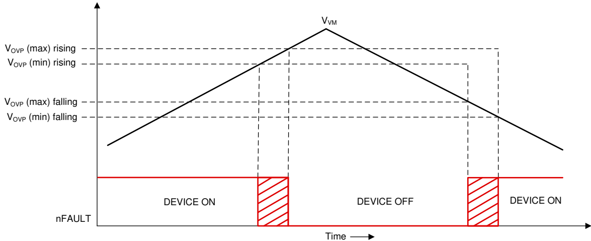
图 7-36. 过压保护
