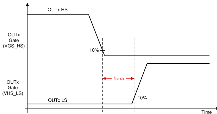
图 7-13. 死区时间
