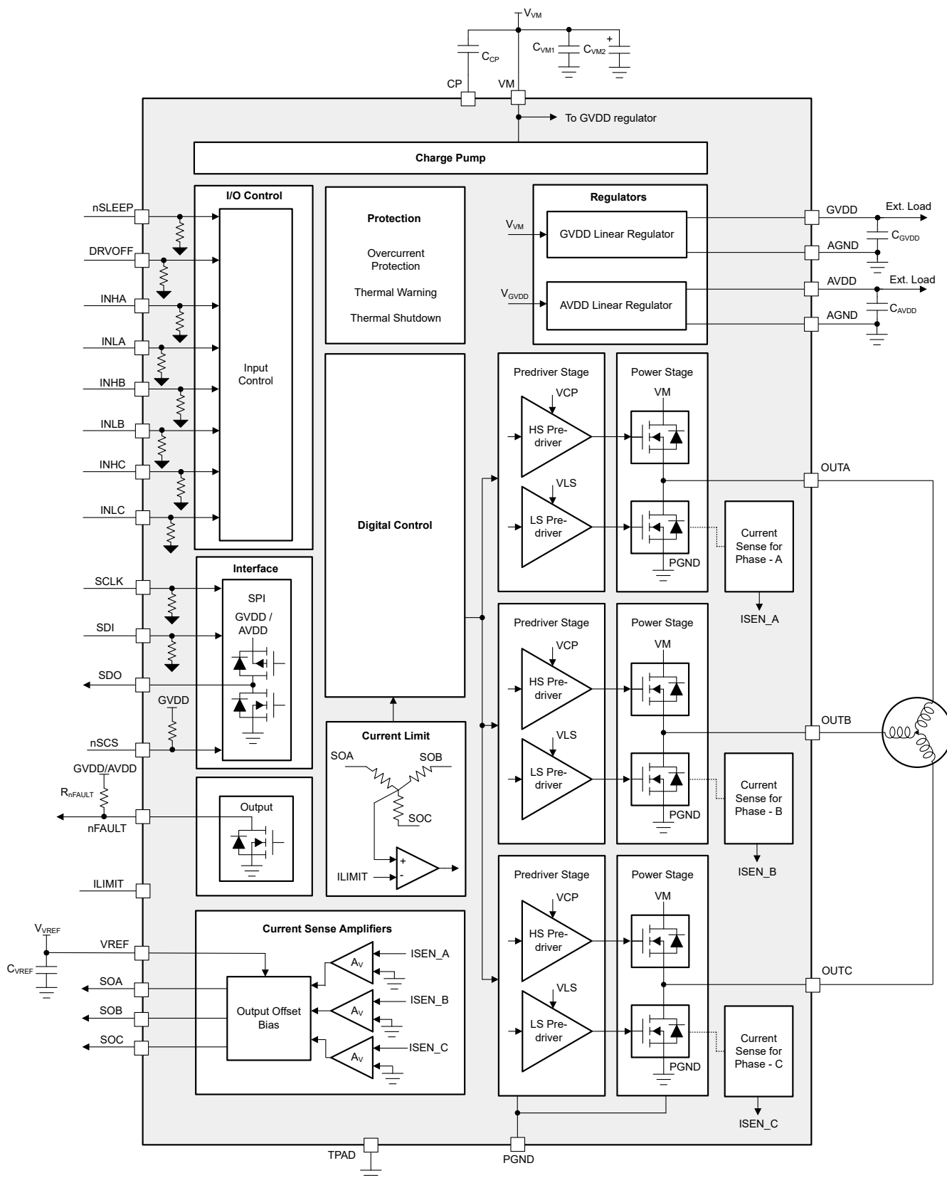
图 7-1 DRV8376S 方框图
