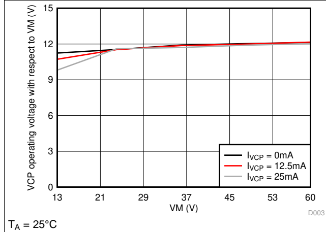
图 4. VCP w.r.t VM over VM voltage > 13 V
