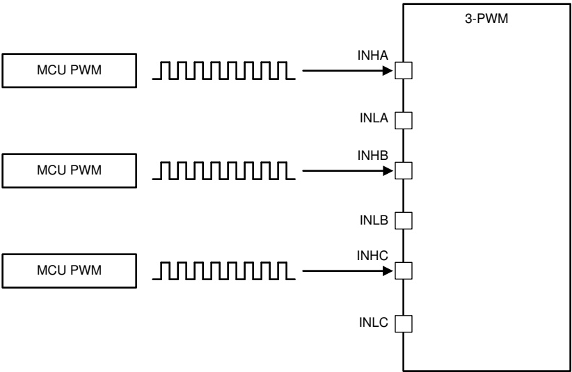
图 9. 3-PWM Mode
