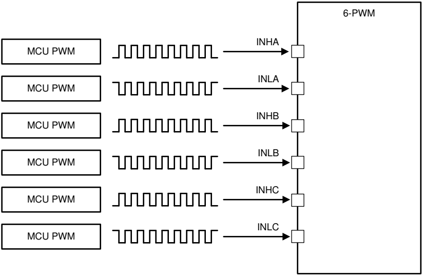
图 8. 6-PWM Mode
