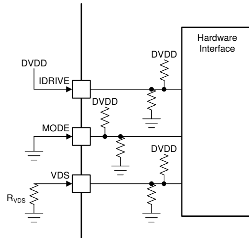
图 17. Hardware Interface
