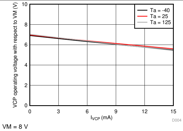
图 5. VCP w.r.t VM over output load I_{VCP}
