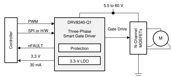
简化原理图
