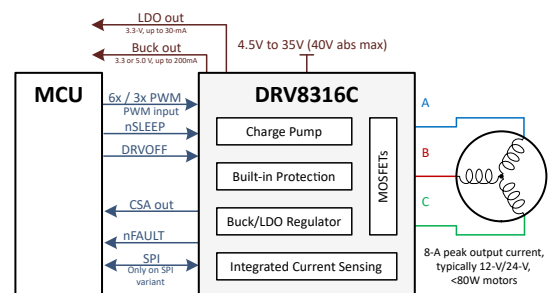
简化原理图
