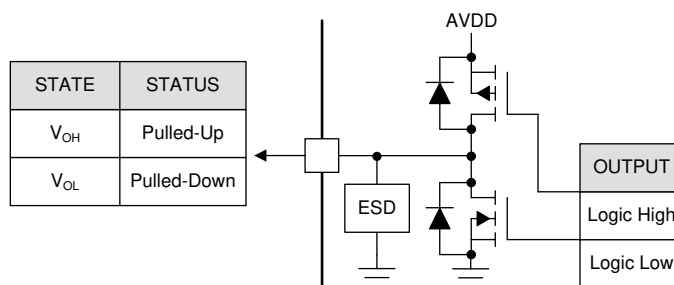
图 8-25. Push Pull
