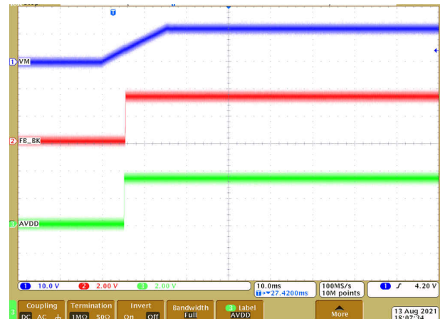
图 9-7. Power management
