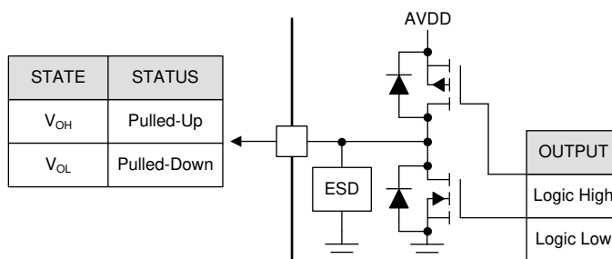
图 8-25. Push Pull
