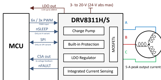
DRV8311H/S 简化版原理图
