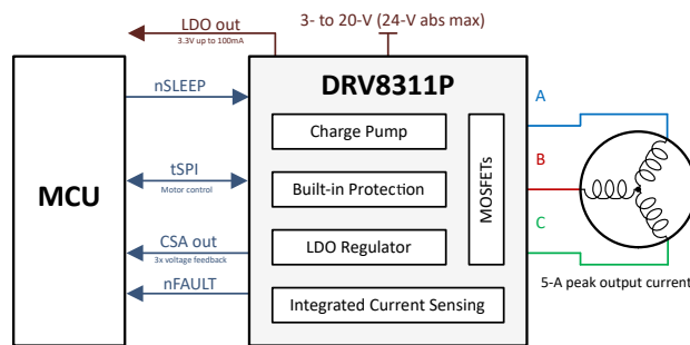
DRV8311P 简化版原理图
