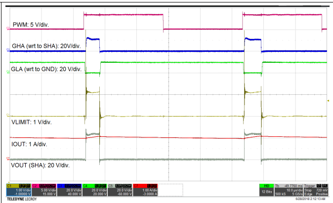
图 38. VLIMIT Operation
