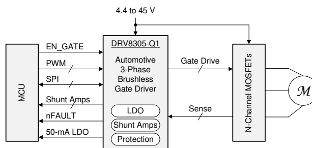
简化原理图
