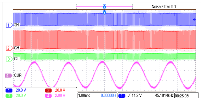
图 8. Motor Spinning 4000 RPM
