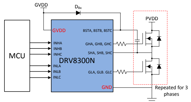
DRV8300N 的简化原理图
