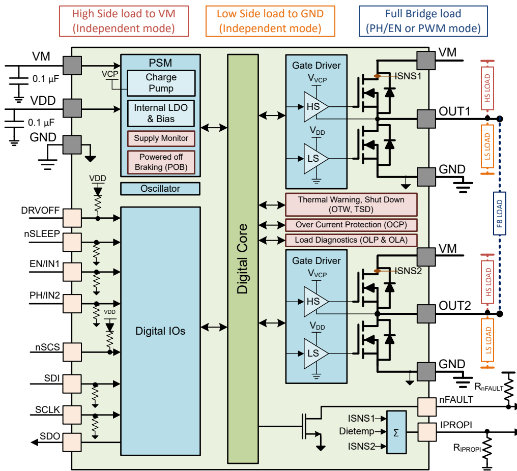
图 7-2. 功能方框图 - SPI 型号
