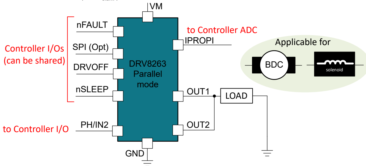
图 9-1. 插图展示了 DRV8263-Q1 处于 PWM 或 PH/EN 模式下的全桥拓扑
