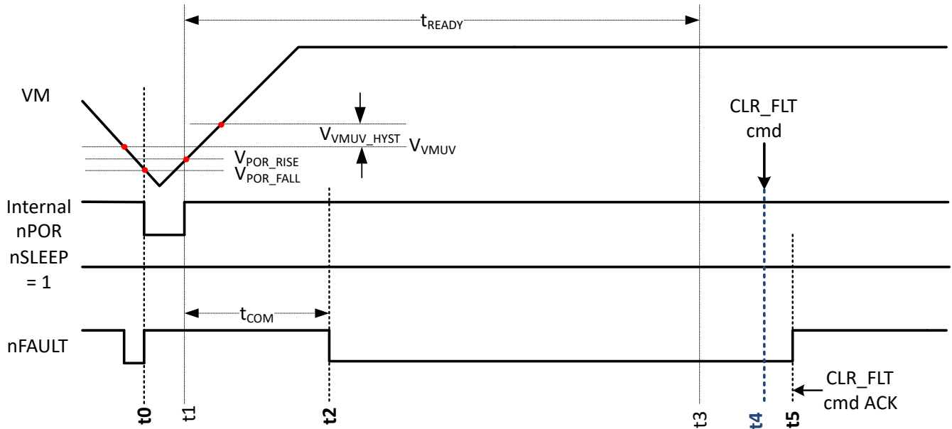
图 6-7. 通过 VM 上电至待机状态的转换
