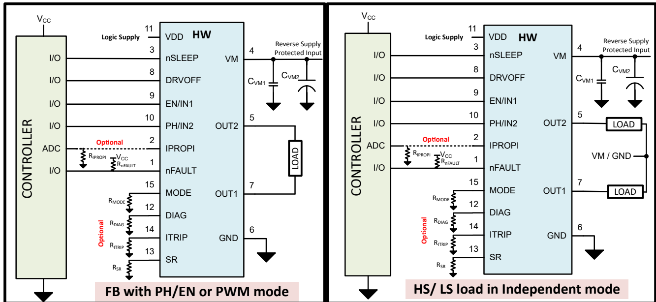
图 9-4. 典型应用原理图 - HW 型号
