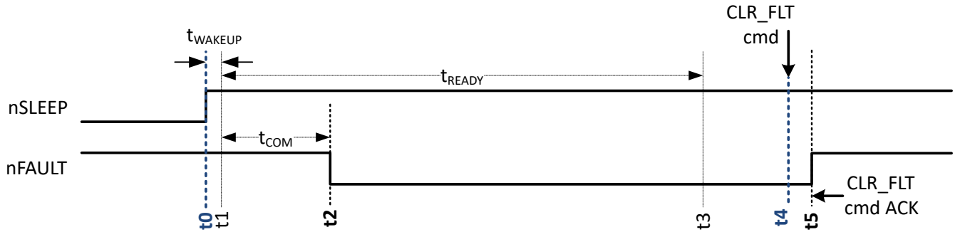
图 6-6. 从休眠状态唤醒后进入待机状态
