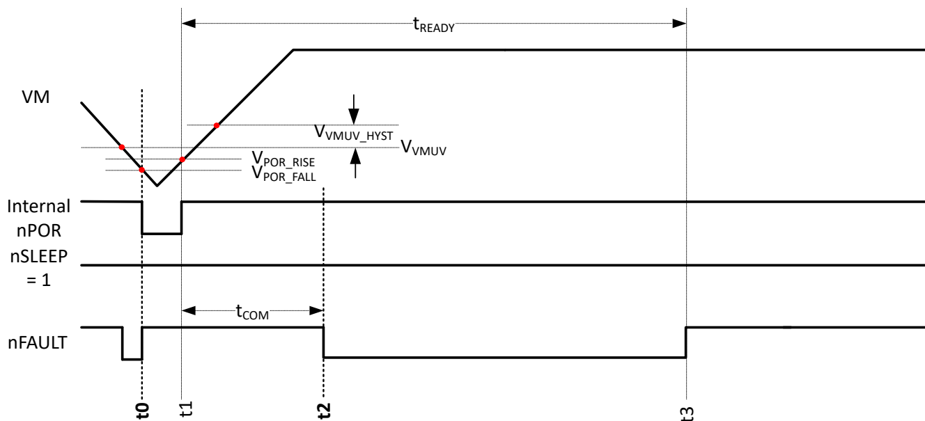
图 6-4. 通过 VM 上电至待机状态
