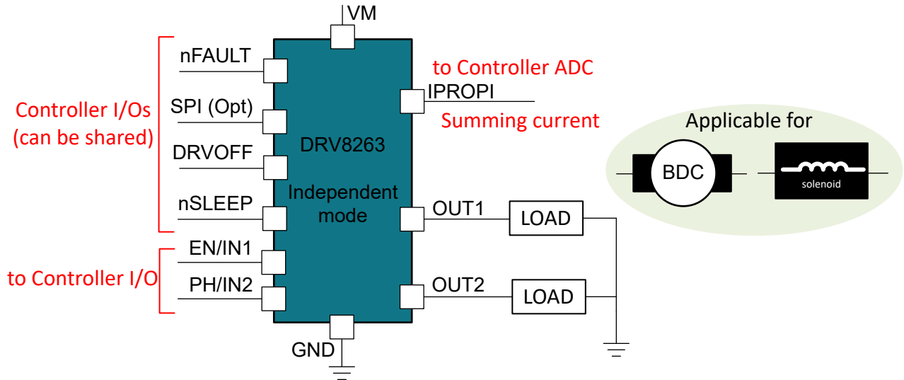
图 9-2. 插图展示了在独立模式下使用 DRV8263-Q1 器件独立驱动两个低侧负载的半桥拓扑
