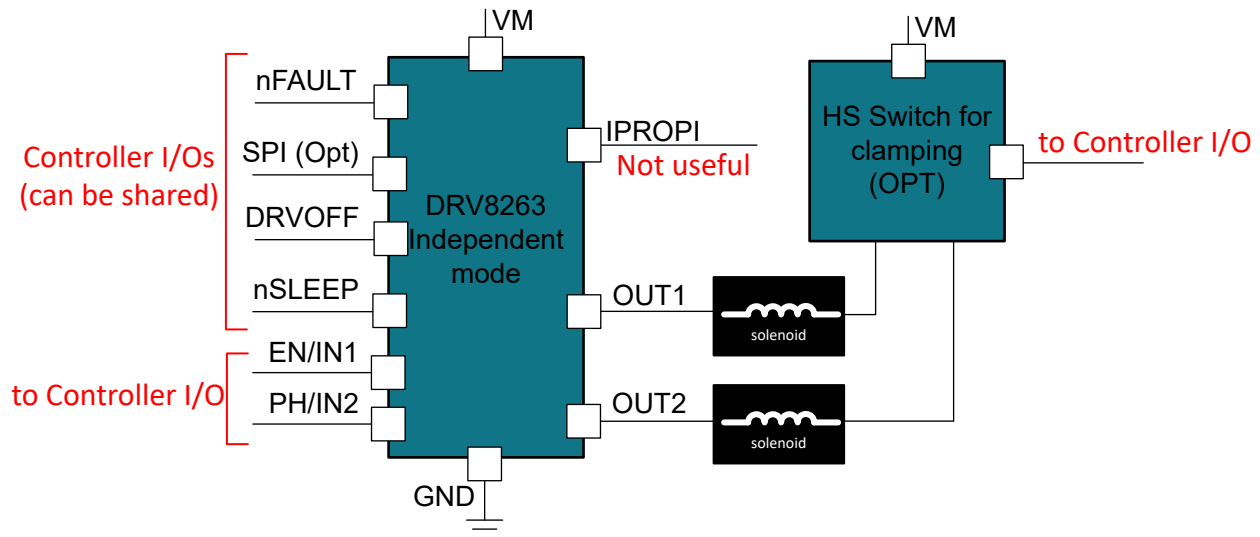
图 9-3. 插图展示了在独立模式下使用 DRV8263-Q1 器件独立驱动两个高侧负载的半桥拓扑
