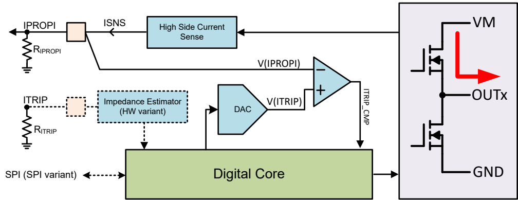
图 7-3. ITRIP 实施
