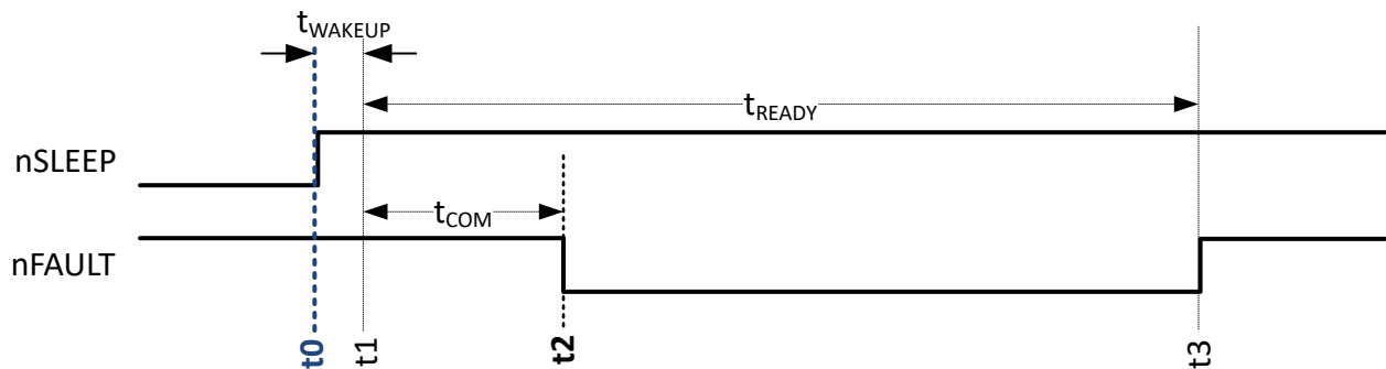
图 6-3. 从休眠状态唤醒后进入待机状态
