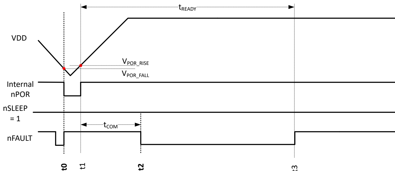
图 6-5. 通过 VDD 上电至待机状态
