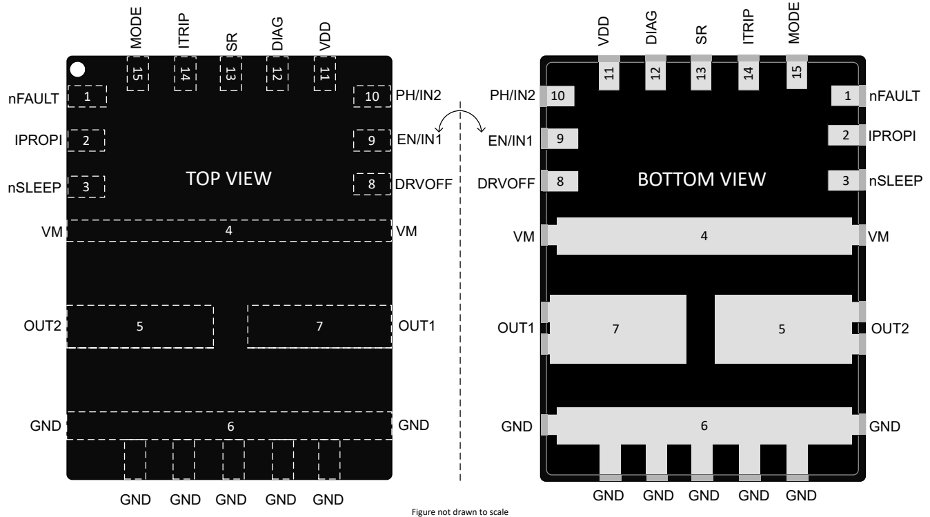
图 5-1. DRV8263H-Q1 型号采用 VQFN-HR(15) 封装
