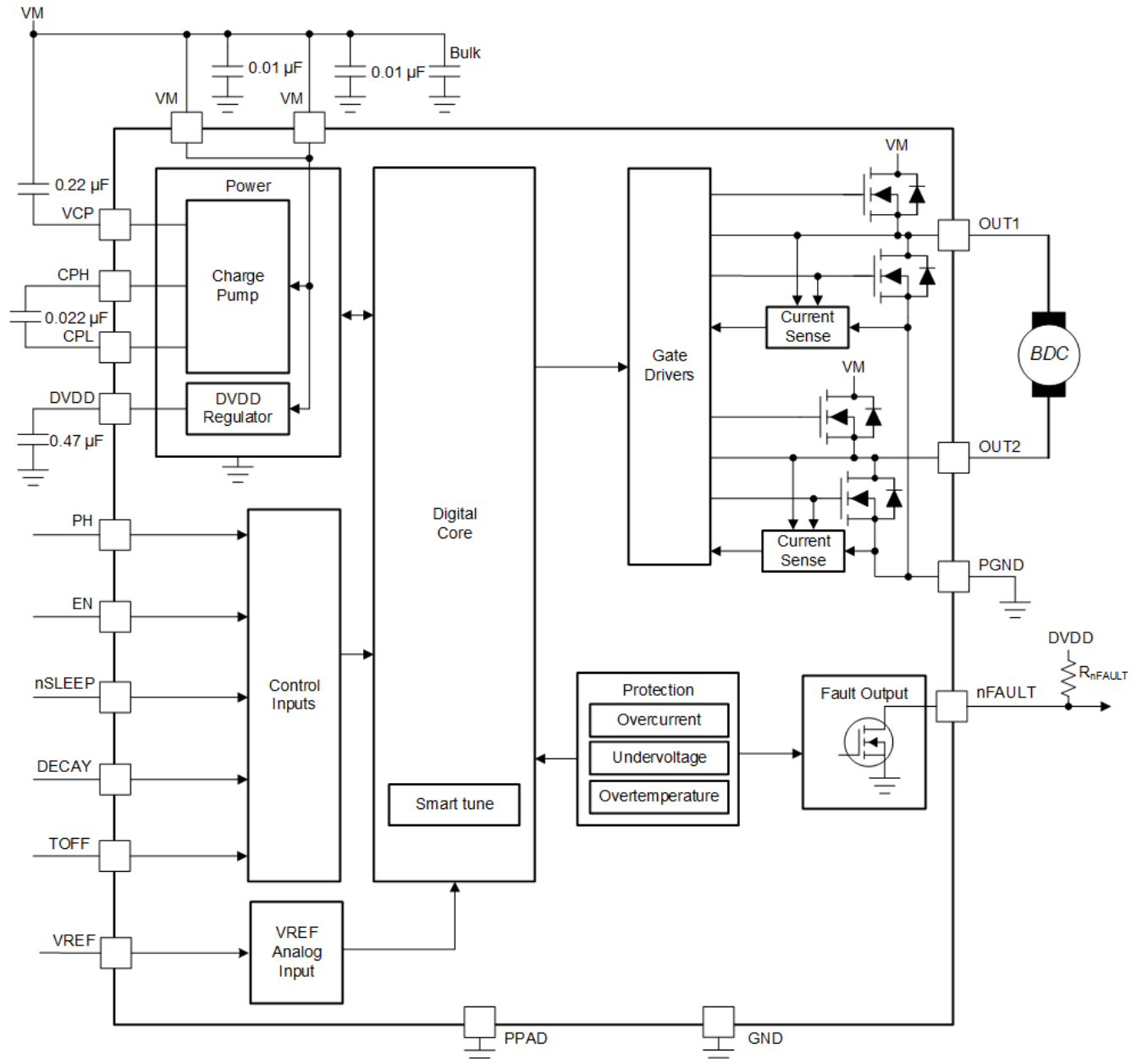
图 7-1. DRV8256E 方框图
