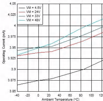
图 6-4. 工作电流与温度间的关系
