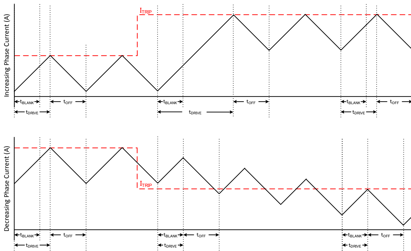
图 7-6. 快速/快速衰减模式
