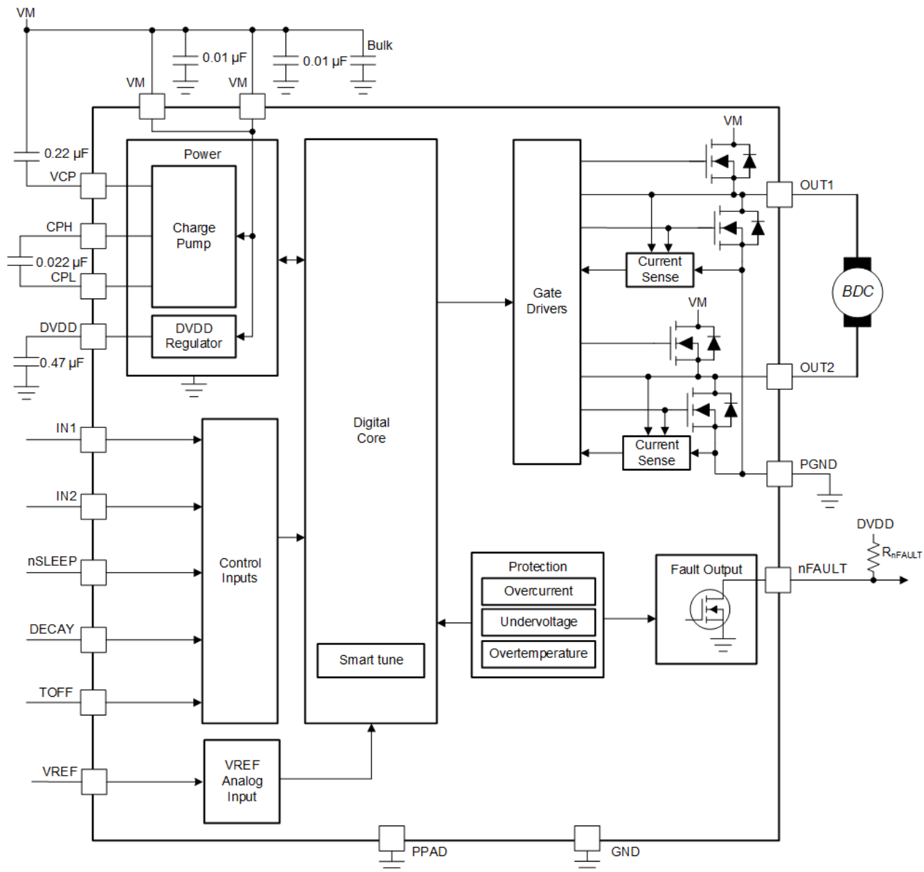
图 7-2. DRV8256P 方框图
