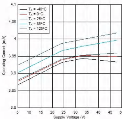
图 6-3. 工作电流与电源电压间的关系
