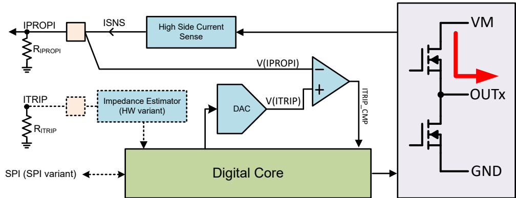
图 8-4. ITRIP 实现
