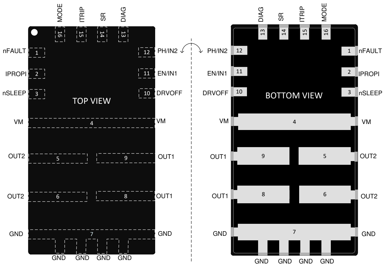
图 6-2. 采用 VQFN-HR(16) 封装的 DRV8244H-Q1 HW 型号
