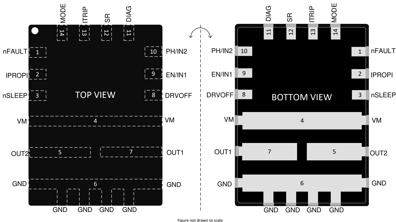
图 6-2. 采用 VQFN-HR (14) 封装的 DRV8243H-Q1 HW 型号
