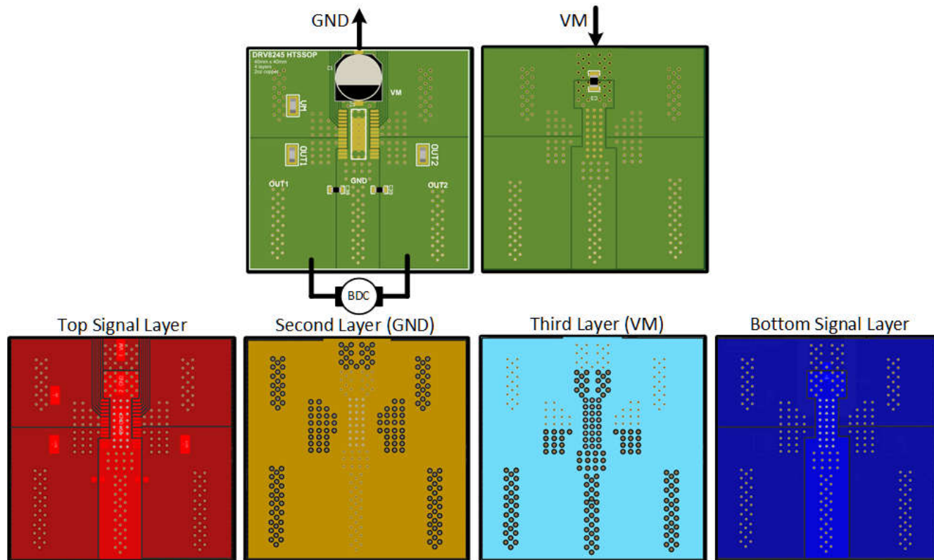
图 9-6. 布局示例：4cm x 4cm x 1.6mm，4 层 PCB
