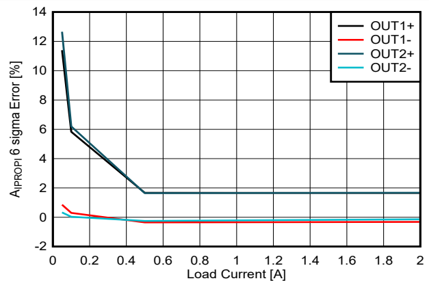
图 6-13. V_{VM} = 13.5V 时 AIPROPI 增益误差与 V 负载电流之间的关系
