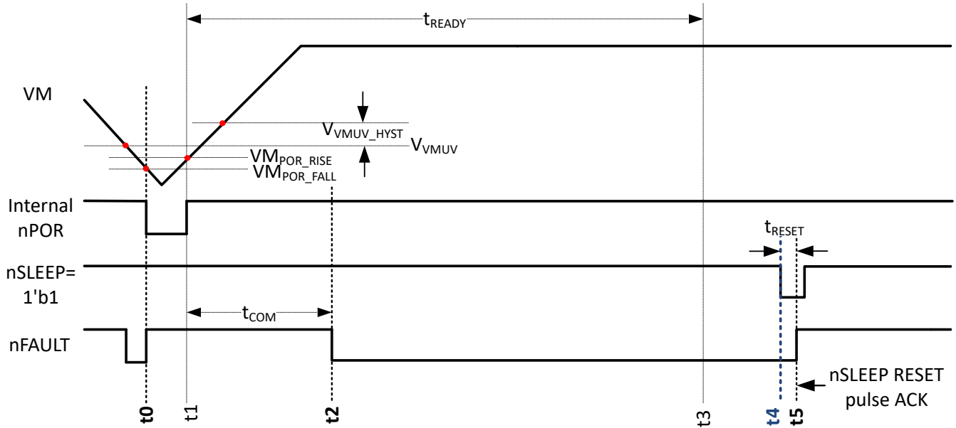
图 6-5. HW 型号从上电至待机状态的转换 (带 ACK 脉冲)
