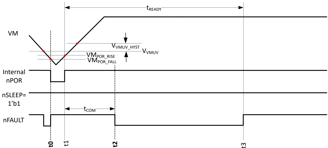
图 6-6. HW 型号从上电至待机状态的转换 (不带 ACK 脉冲)
