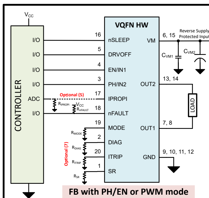
图 9-2. 典型应用原理图 - 采用 VQFN 封装的 HW 型号
