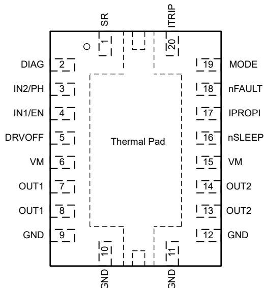
图 5-1. 采用 VQFN (20) 封装的 DRV8242H-Q1 HW 型号
