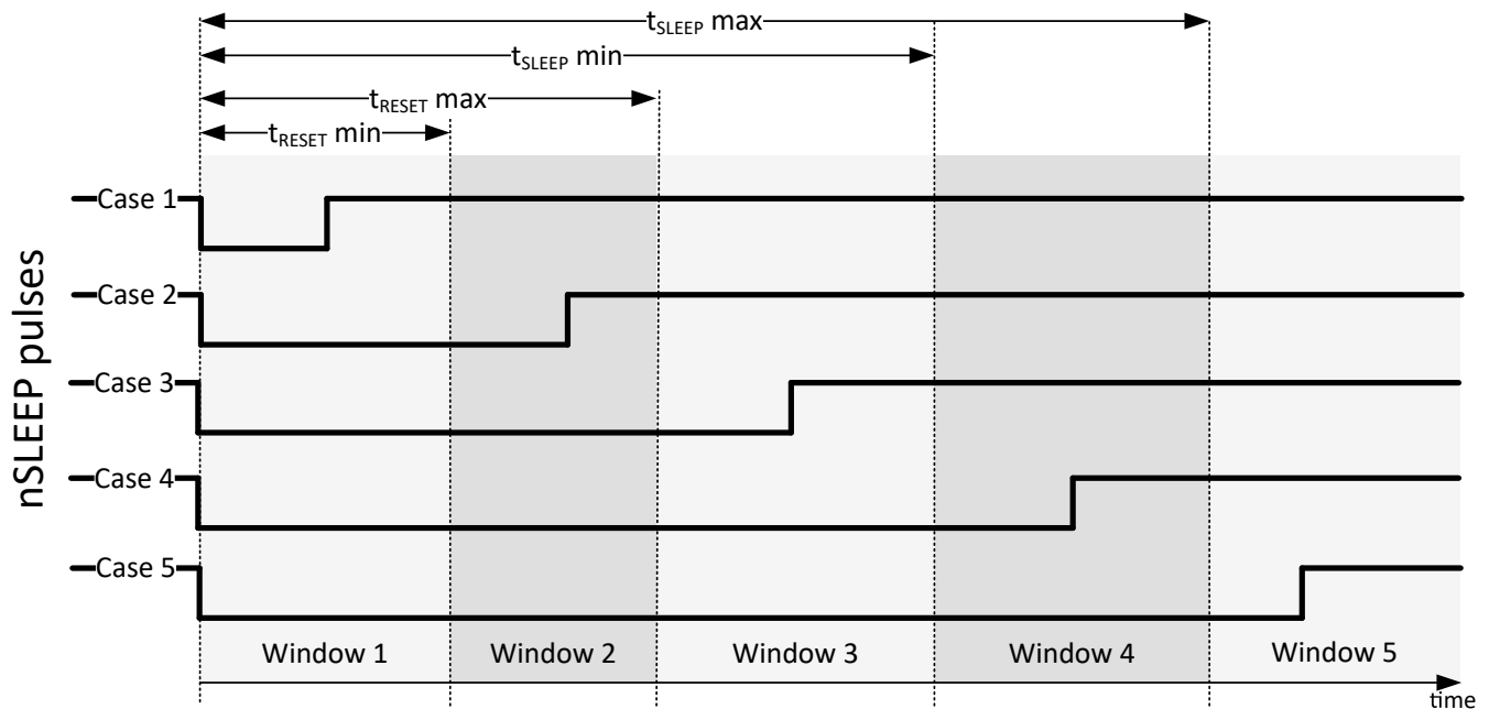
图 7-9. nSLEEP 脉冲场景
