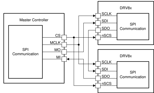
图 7-12. 使用菊花链时的 SPI 操作
