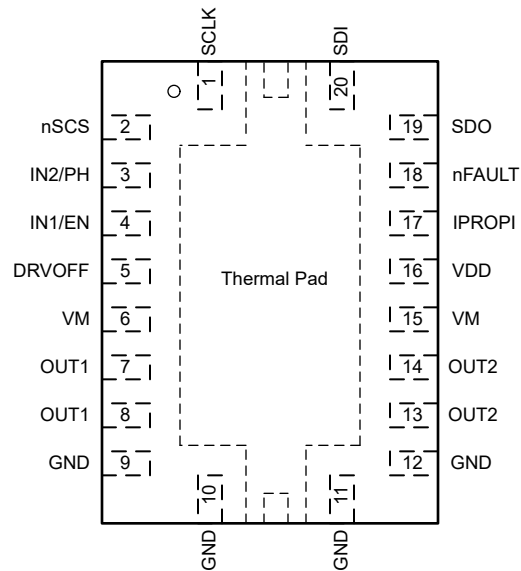
图 5-3. 采用 VQFN (20) 封装的 DRV8242S-Q1 SPI 型号
