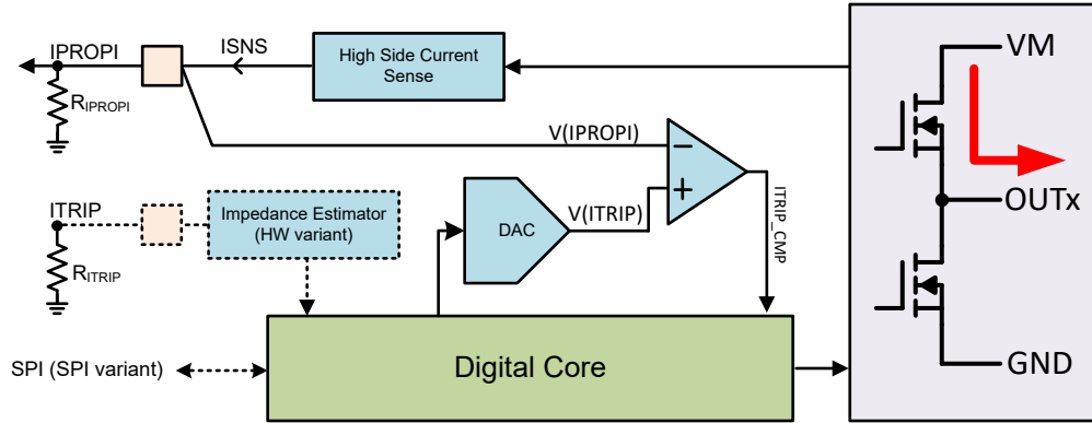
图 7-4. ITRIP 实现
