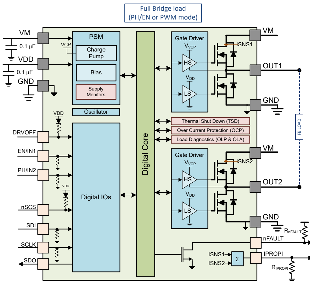
图 7-3. 功能方框图 - SPI (P) 型号
