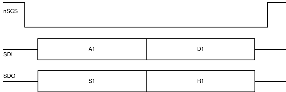
图 7-10. SPI 数据 - 标准“16 位”帧
