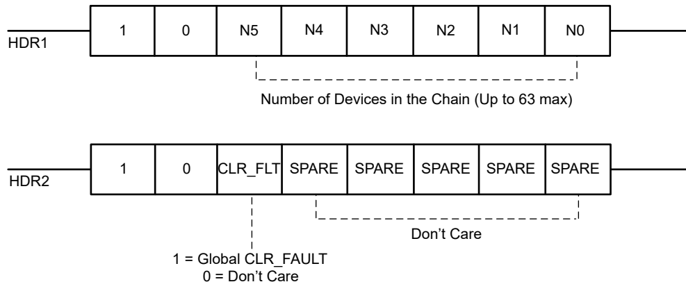
图 7-14. 标头字节
