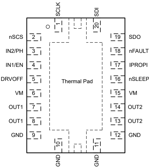
图 5-2. 采用 VQFN (20) 封装的 DRV8242S-Q1 SPI 型号
