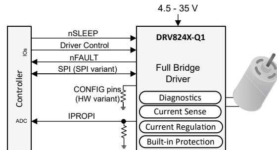
简化原理图
