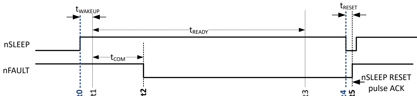
图 6-3. HW 型号从休眠状态唤醒到待机状态的转换 (带 ACK 脉冲)
