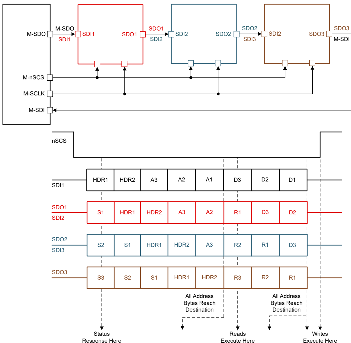
图 7-13. 菊花链 SPI 操作
