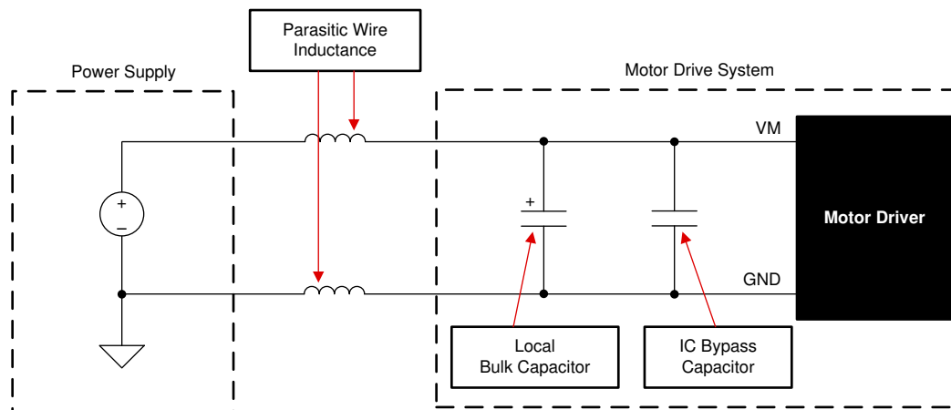
图 9-5. 带外部电源的电机驱动系统设置示例
