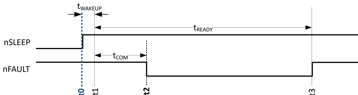
图 6-4. HW 型号从休眠状态唤醒到待机状态的转换 (不带 ACK 脉冲)
