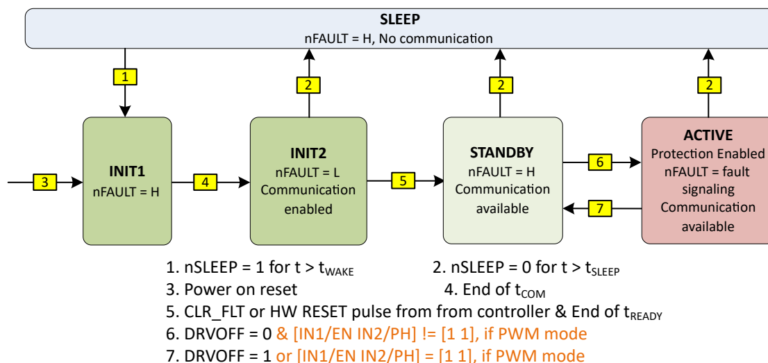
图 7-8. 说明性状态图
