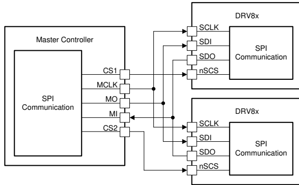
图 7-11. 不使用菊花链时的 SPI 操作
