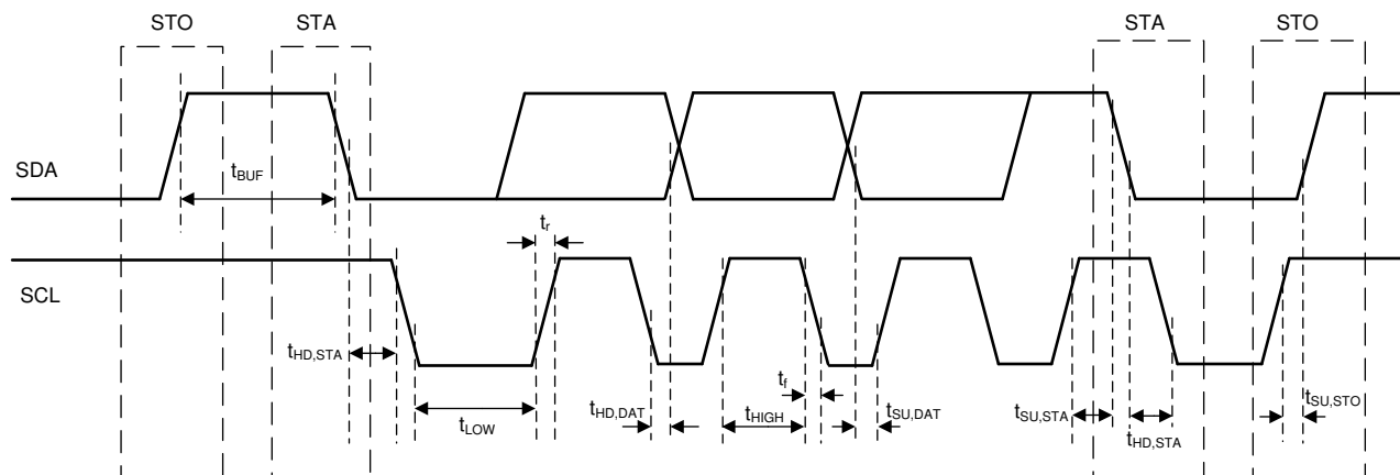
图 6-2. I²C 时序图
