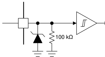
图 8-14. 逻辑电平输入
