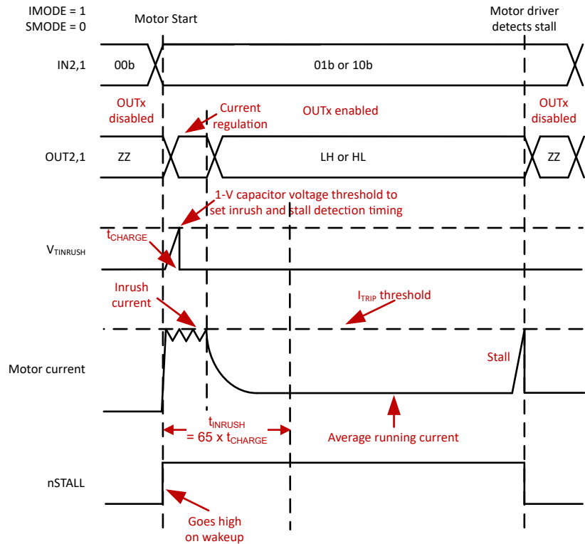
图 9-4. 硬件失速检测的示例时序图
