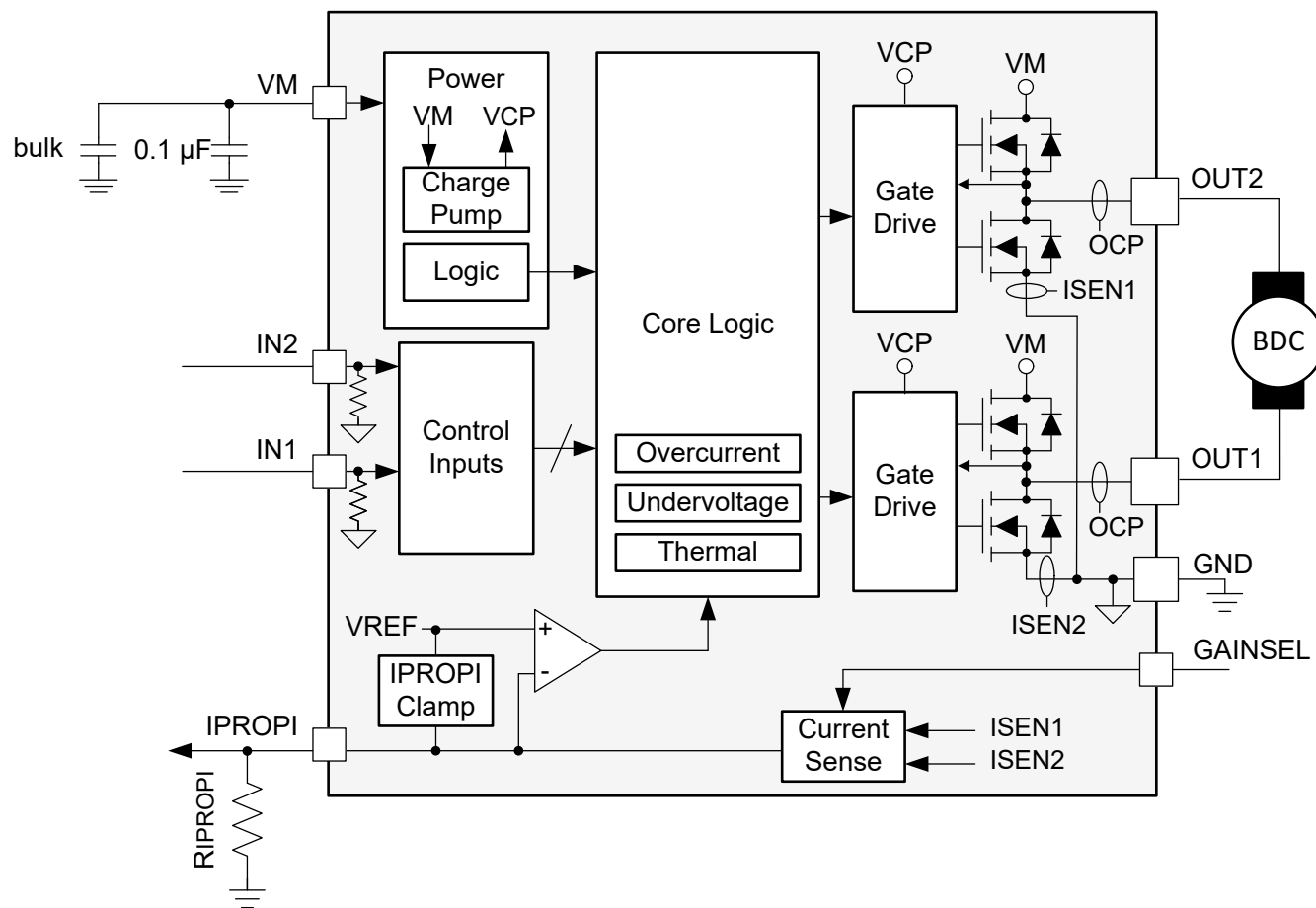
图 8-1. DRV8213 采用 WSON (DSG) 封装，具有单电源引脚
