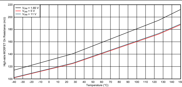
图 7-2. 高侧 MOSFET 导通电阻 (DSG 封装)
