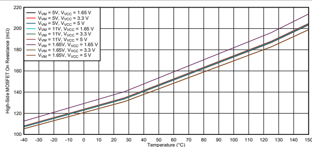
图 7-6. 高侧 MOSFET 导通电阻 ( RTE 封装 )
