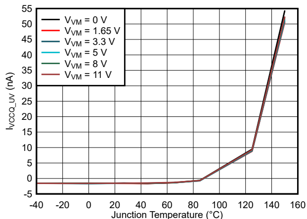
图 7-10. VCC 为低电平时的 VCC 电源电流 ( I_{VCCQUV} ) 与结温 ( T_J )
