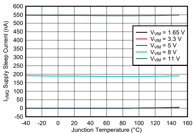
图 7-18. 休眠电流 ( I_{VMQ} ) 与结温 ( T_J )
