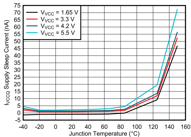
图 7-4. 休眠电流 ( I_{VCCQ} ) 与结温 ( T_J )
