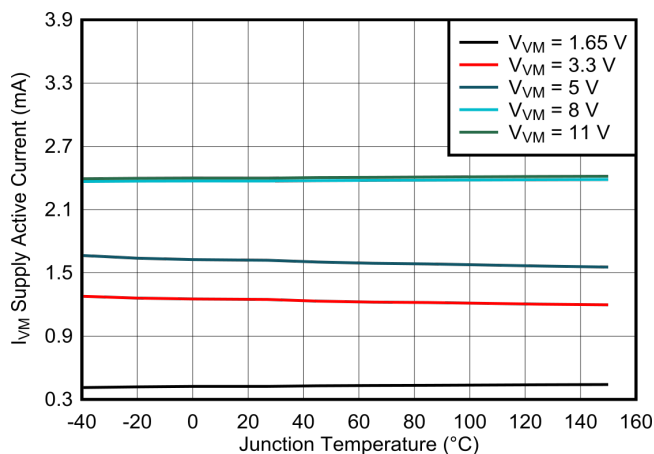
图 7-20. 有效电流 ( I_{VM} ) 与结温 ( T_J )
