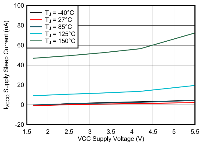
图 7-3. 休眠电流 ( I_{VCCQ} ) 与电源电压 ( V_{VCC} )
