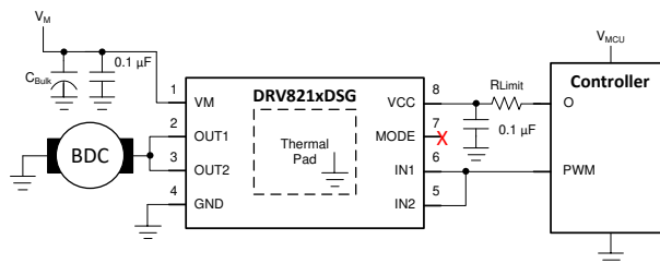
图 9-10. 半桥模式用作输出并联的高侧驱动器
