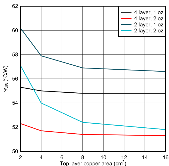
图 9-32. WSON、结至电路板特征参数与铜面积
