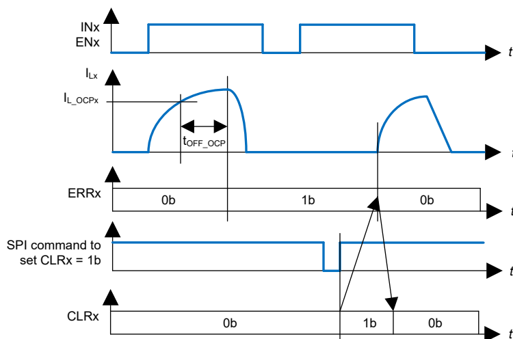
图 7-14. 过流锁闭
