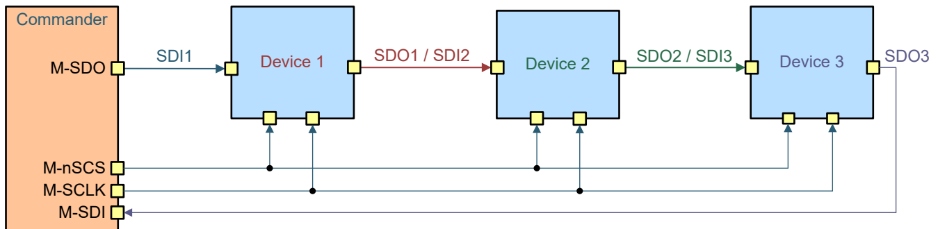
图 7-24. 菊花链配置
