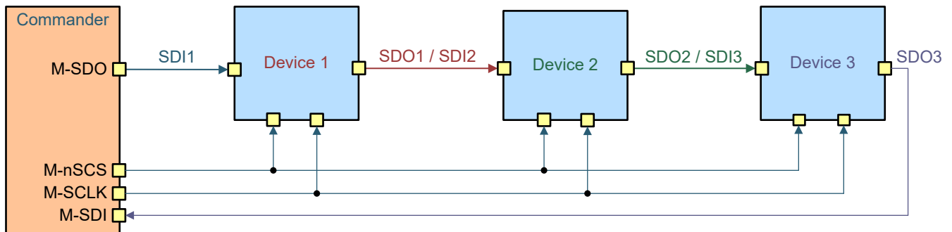
图 7-24. 菊花链配置
