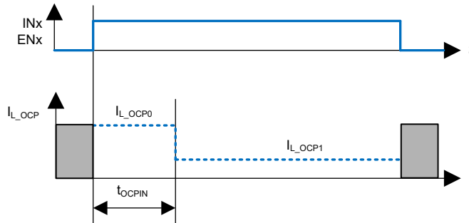
图 7-13. 过流阈值
