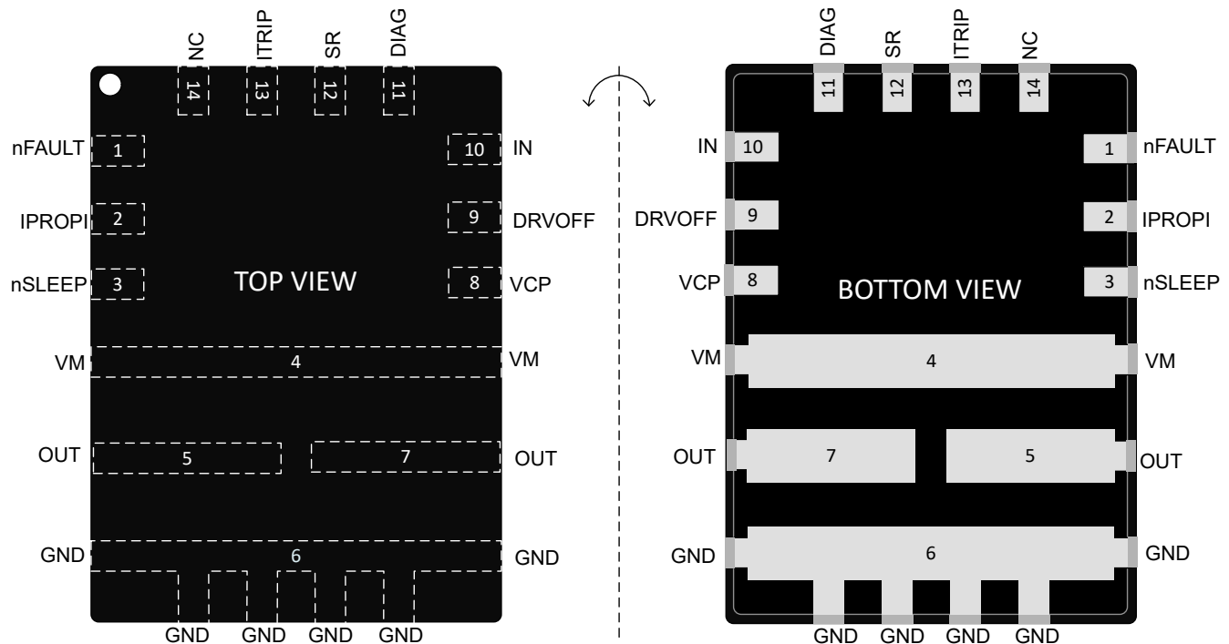
图 5-1. 采用 VQFN-HR (14) 封装的 DRV8143H-Q1 HW 型号
