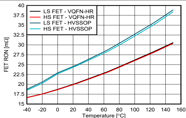
图 6-11. V_{VM} = 13.5V 时 R_{HS\_ON} 和 R_{LS\_ON} 与温度之间的关系
