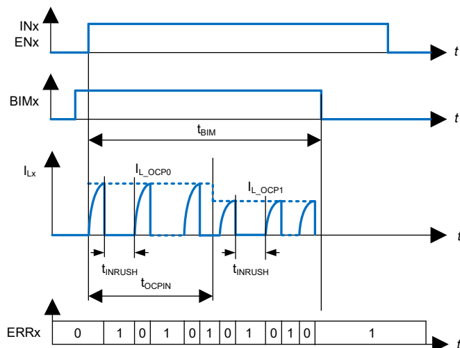
图 7-11. 灯泡浪涌模式 (BIM) 运行
