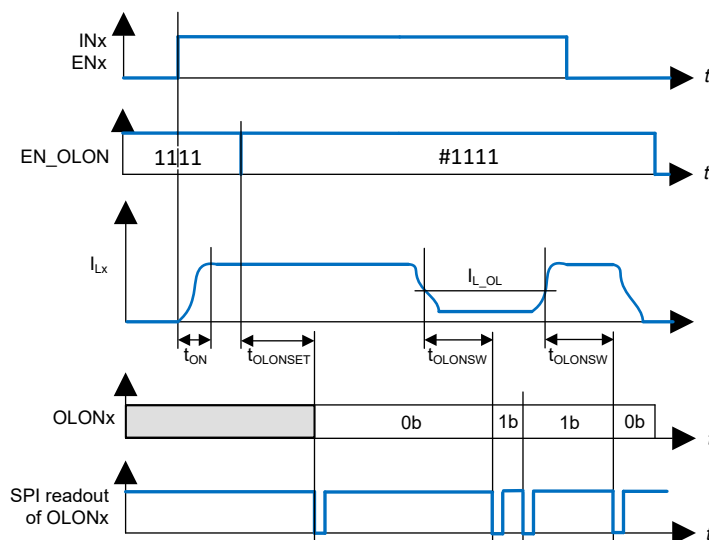
图 7-22. 导通时序时的开路负载 (直接通道诊断)
