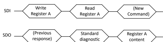
图 7-28. 寄存器内容发送回微控制器
