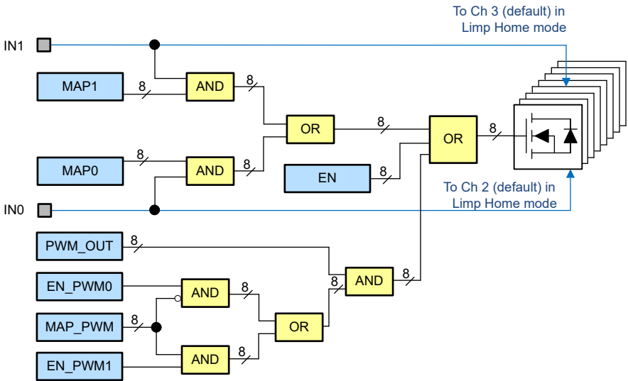
图 7-12. PWM 发生器映射
