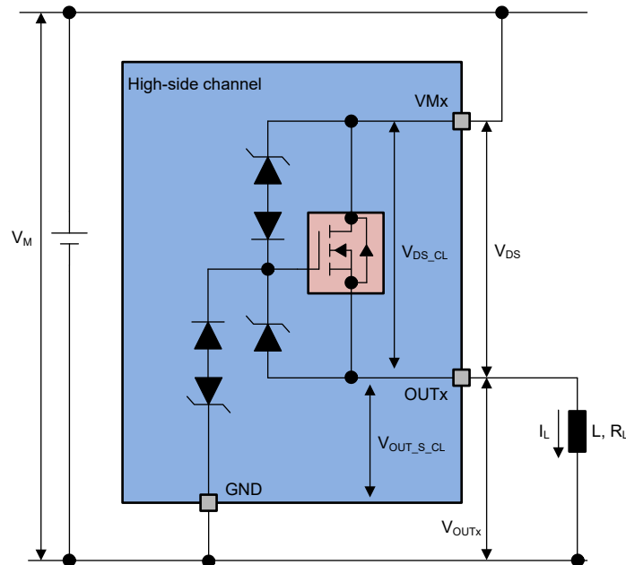
图 7-10. 高侧通道的输出钳位
