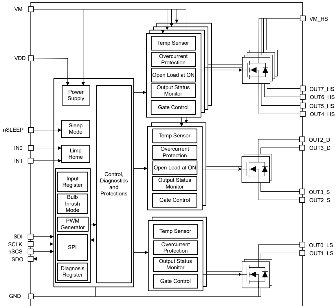
图 7-1. DRV81242-Q1 功能方框图
