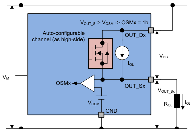
图 7-19. 输出状态监控 - 自动可配置通道为高侧
