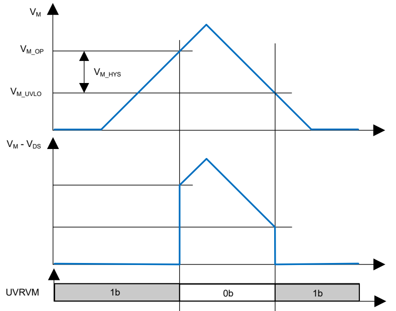
图 7-13. V_M 欠压行为
