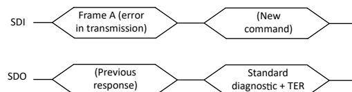
图 7-29. 传输出错之后的响应
