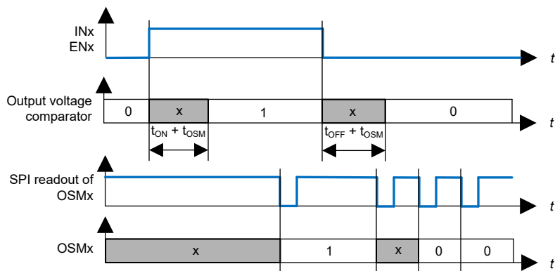
图 7-17. 输出状态监控时序
