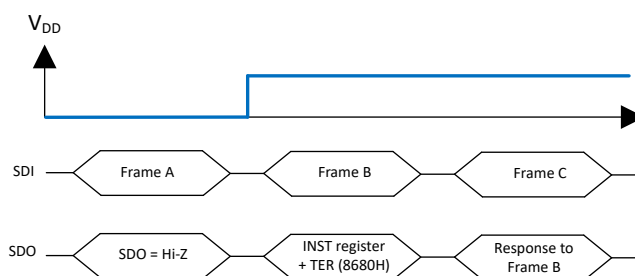
图 7-30. 退出 V_{DD} 上电复位后的响应
