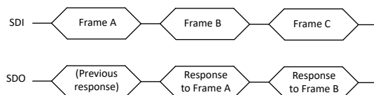
图 7-27. SPI 通信期间 SDI 和 SDO 之间的关系
