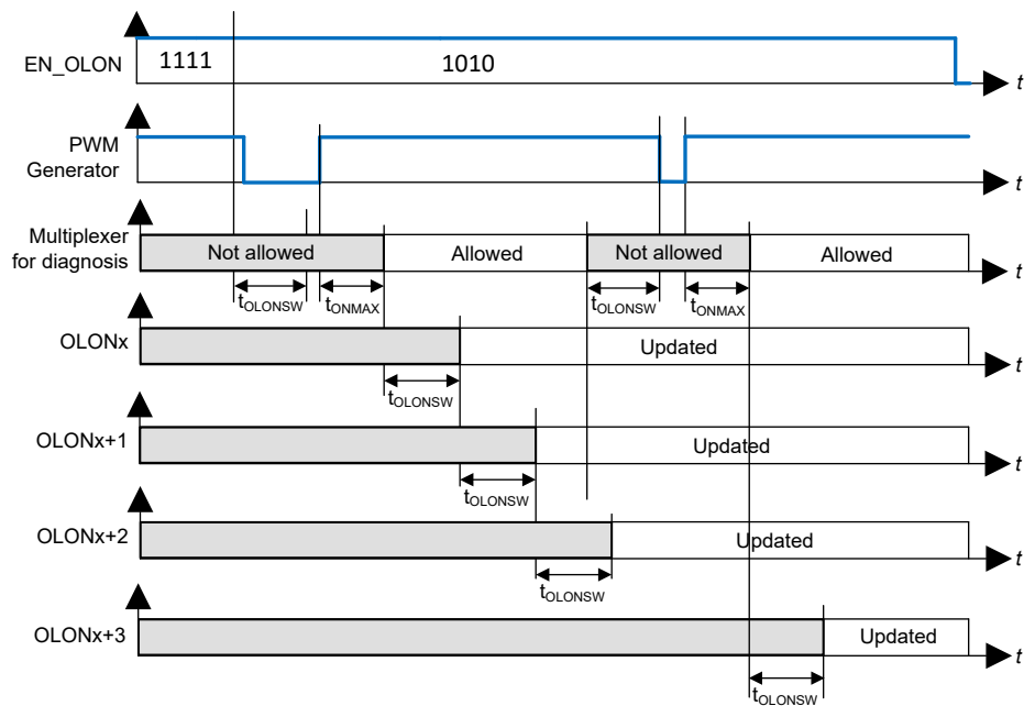
图 7-24. 导通时序时的负载开路 ( 诊断环路 - 由内部 PWM 发生器驱动通道 )
