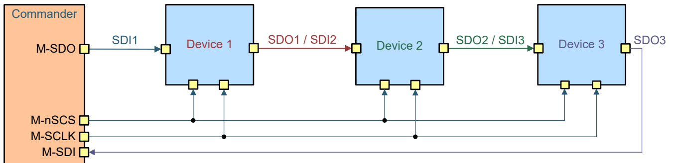
图 7-26. 菊花链配置
