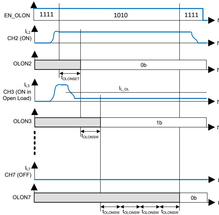
图 7-23. 导通时序时的负载开路 ( 诊断环路 - 由微控制器驱动通道 )
