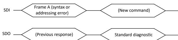
图 7-31. 命令语法错误后的响应
