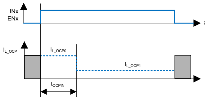
图 7-14. 过流阈值
