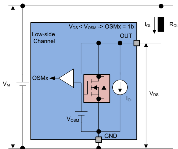
图 7-18. 输出状态监控 - 低侧通道
