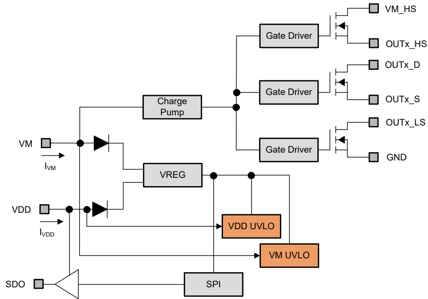
图 7-3. 内部电源架构
