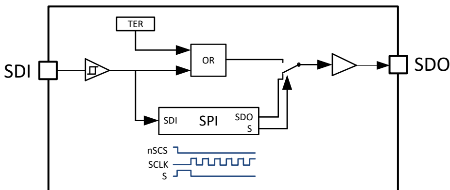
图 7-25. TER 位组合逻辑
