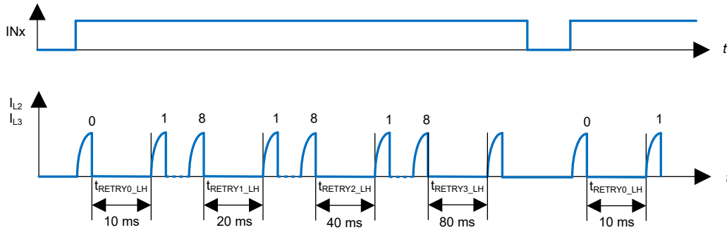
图 7-16. 在跛行回家模式下重新启动计时器
