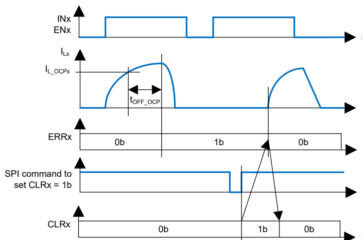
图 6-11. 过流锁闭
