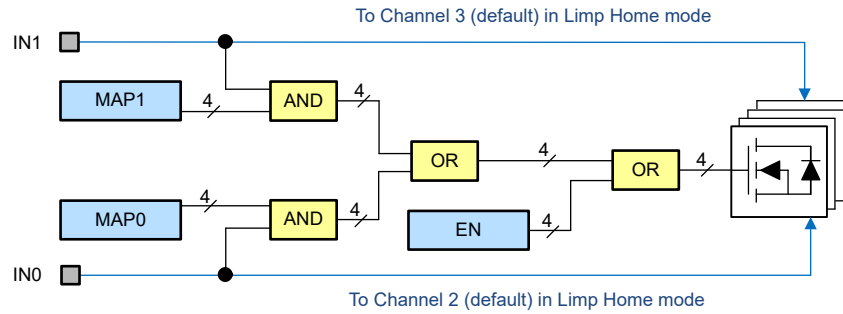
图 6-2. 输入映射
