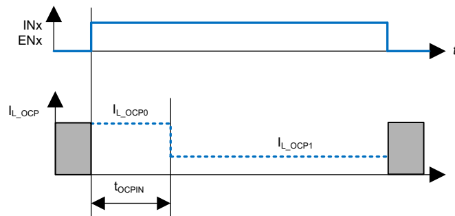
图 6-10. 过流阈值
