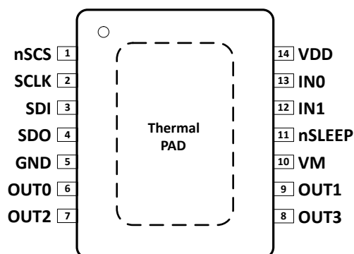
图 4-1. 14 引脚 HTSSOP (PWP) 顶视图
