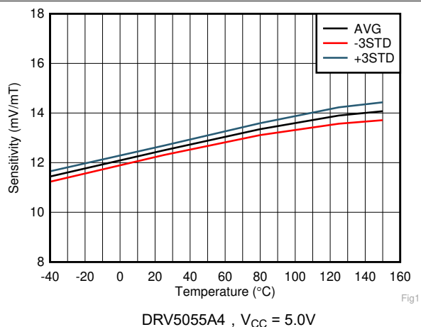
图 5-13. 灵敏度与温度之间的关系
