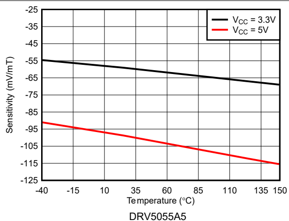
图 5-14. 灵敏度与温度之间的关系
