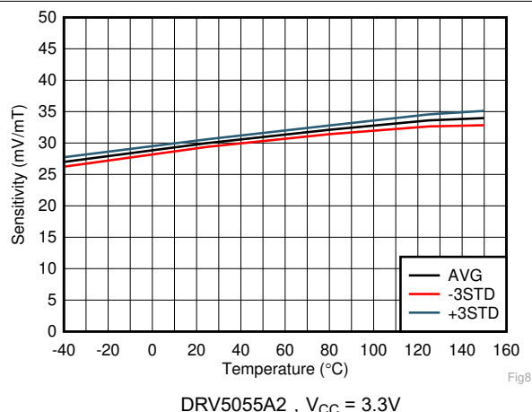
图 5-8. 灵敏度与温度之间的关系
