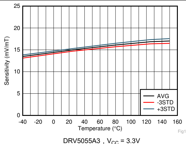
图 5-10. 灵敏度与温度之间的关系
