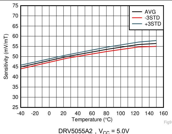
图 5-9. 灵敏度与温度之间的关系
