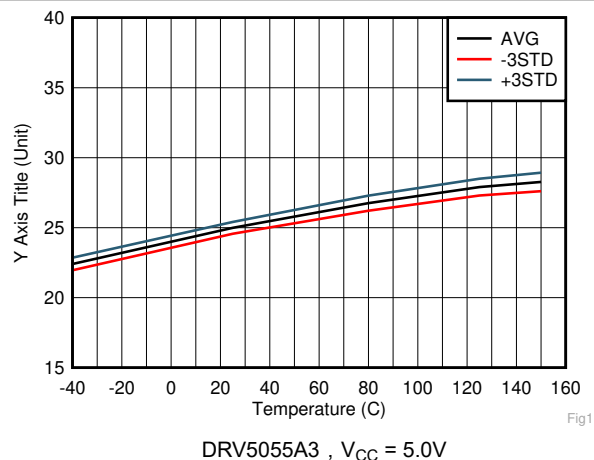
图 5-11. 灵敏度与温度之间的关系
