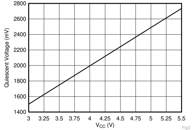
图 5-2. 静态电压与电源电压之间的关系
