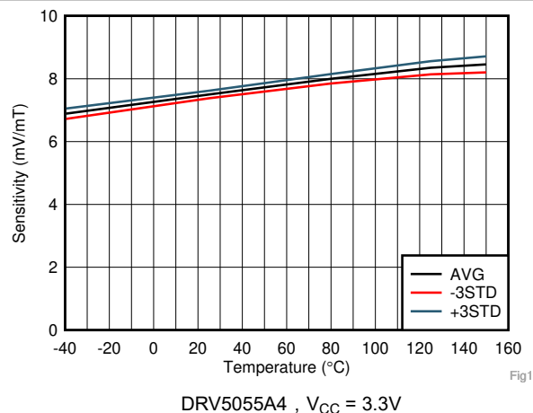
图 5-12. 灵敏度与温度之间的关系
