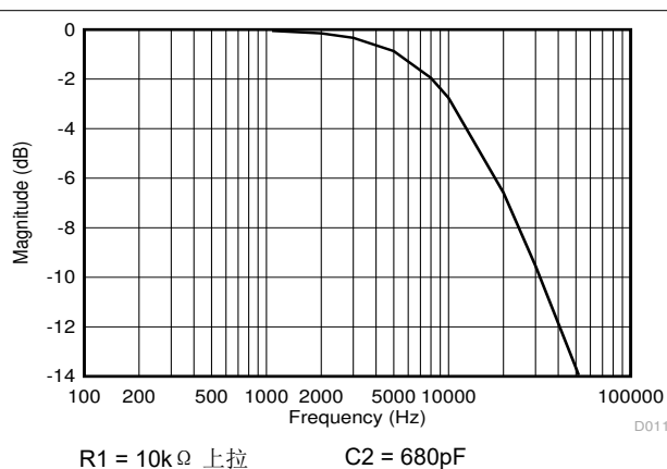
图 8-5. 低通滤波
